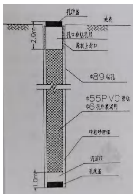
图 8-1 地下水采样监测井施工图
