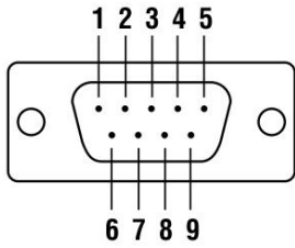
RS-232 DB-9(Male)
