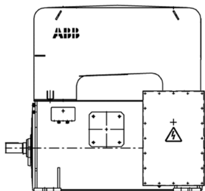
Code I: IM B3 Code II: IM 1001 Horizontal foot mounted
