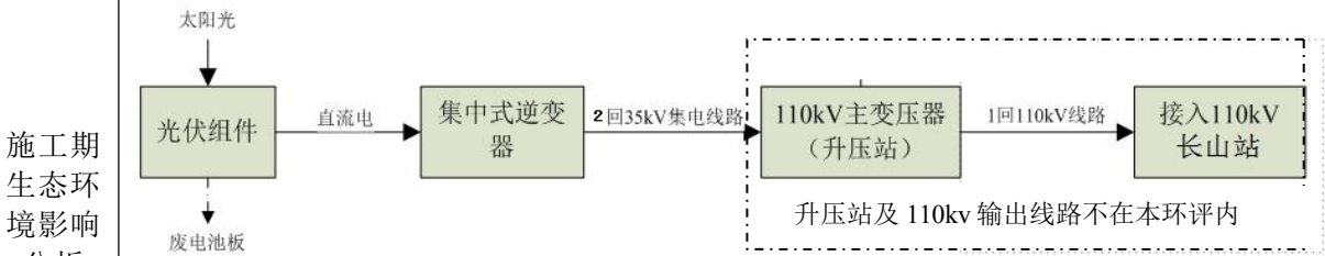
图 4-1b 营运期工艺流程及产污环节
