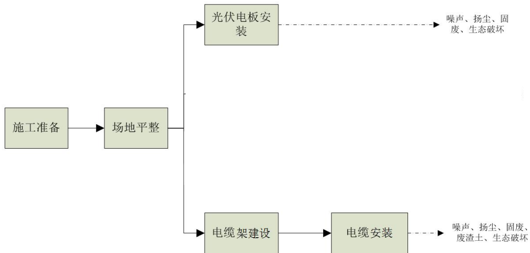
图 4-1a 施工期工艺流程及产污环节
