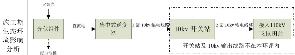
图 4-1b 营运期工艺流程及产污环节
