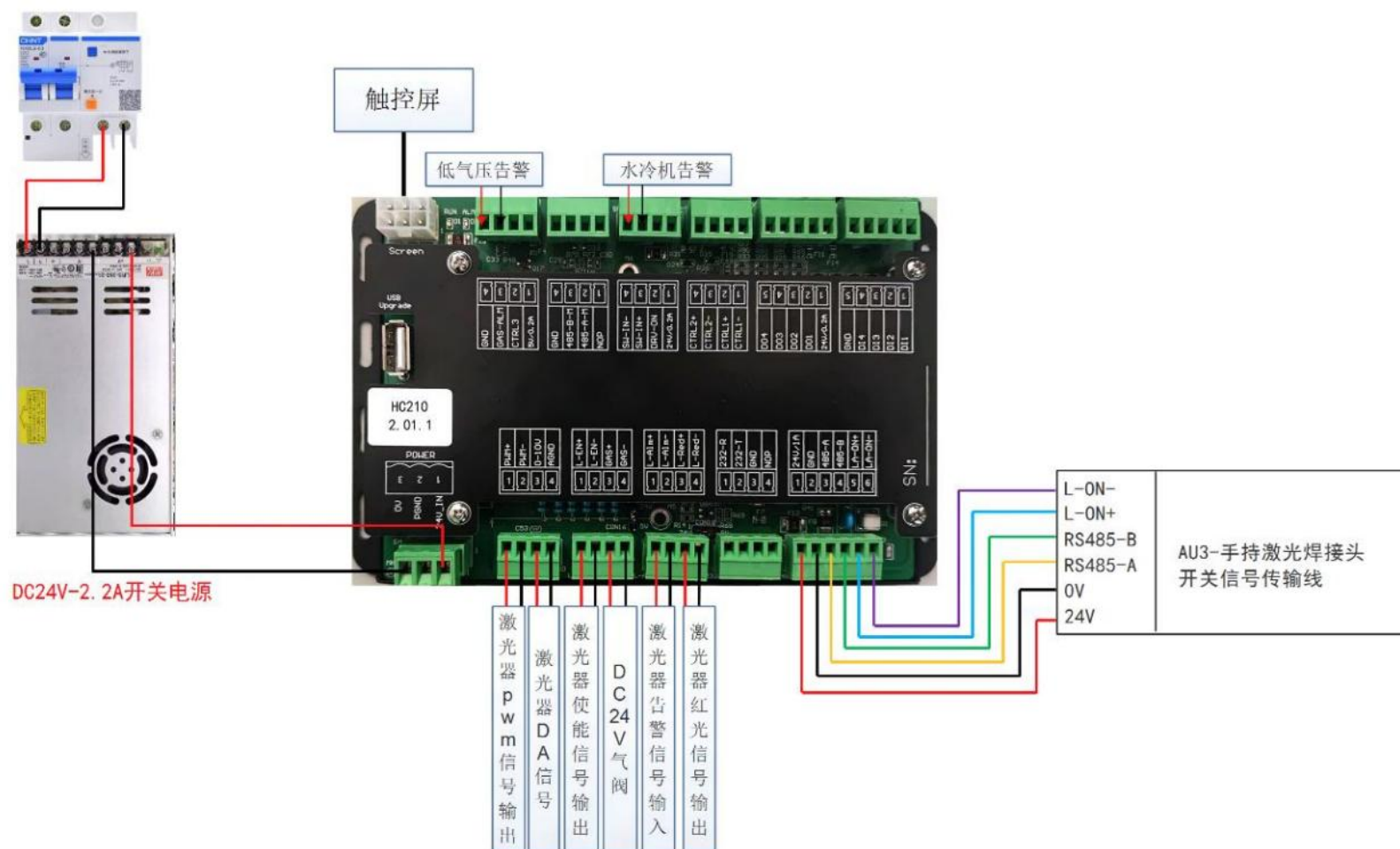
HC210手持清洗系统接线图
