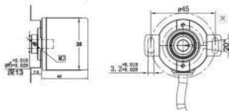
38mm 外径 6/8mm 孔径 13mm 孔深 轴向出线可选
