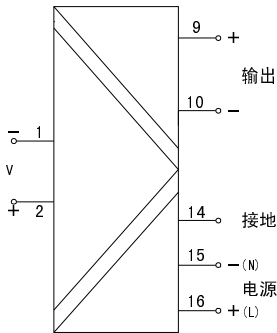
单路电压输入-单输出
