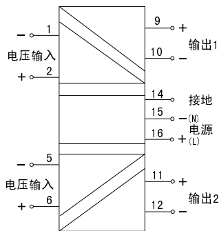
双路电压输入-双输出
