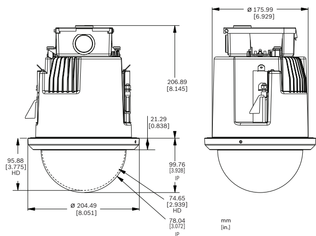
AUTODOME 7000 尺寸 - 嵌入天花板式
