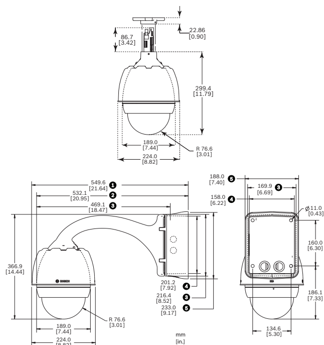
AUTODOME 7000 尺寸 - 吊装式、管道式
