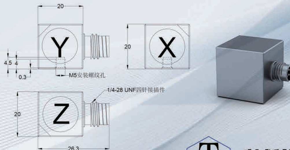
外形图:
