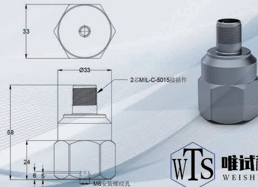
外形图:
