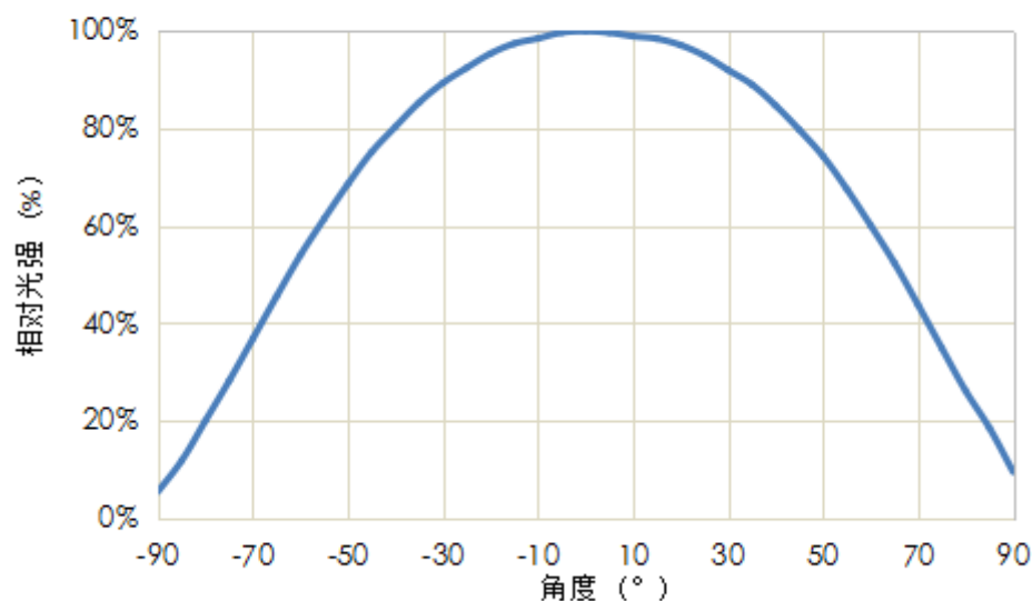
相对光强 vs 角度 I_f=1000\text{mA}
