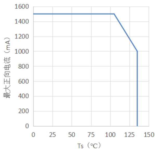
最大电流 VS T s 温度
