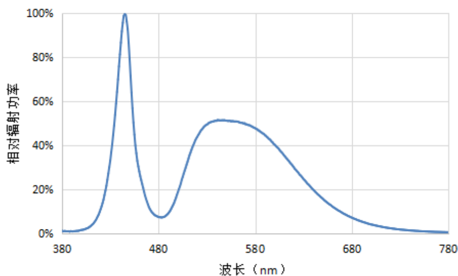
相对辐射功率 VS 波长 I_f=1000\text{mA}
