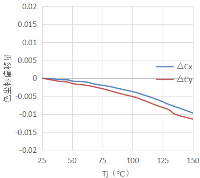
色坐标偏移量 VS T j 温度 I f =1000mA
