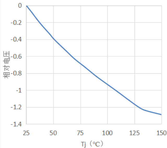
相对电压 VS T j 温度 I f =1000mA
