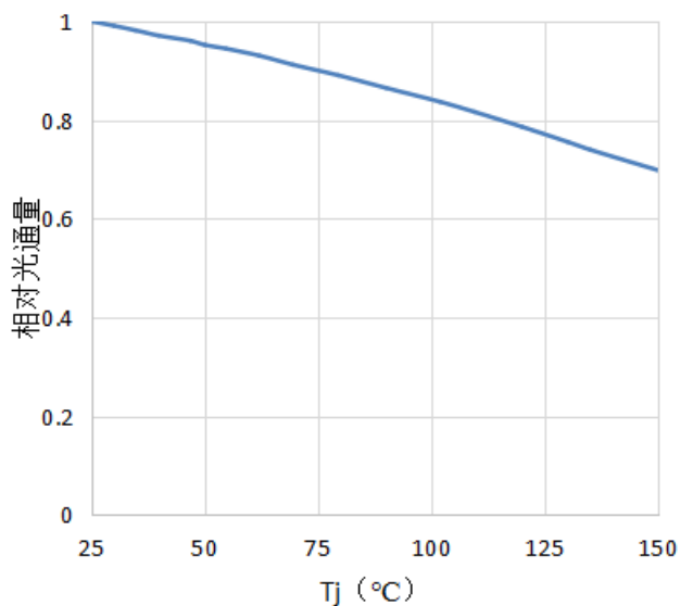
相对光通量 VS T j 温度 I f =1000mA
