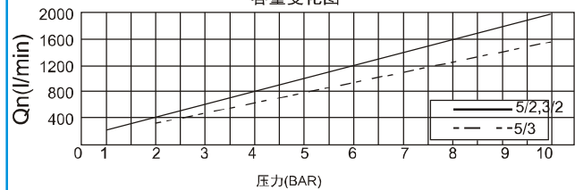
容量变化图
