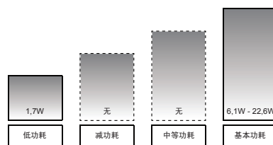
功耗等级 - 冷态式线圈功耗 (W)
