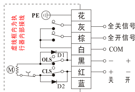
G型:直流控制电路(无源触点)
