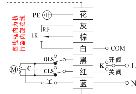
C型:带1K电位器
