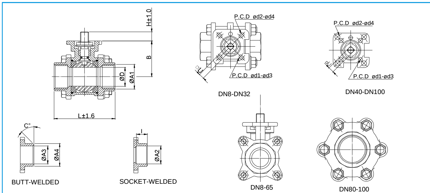
外形尺寸 Dimensions
