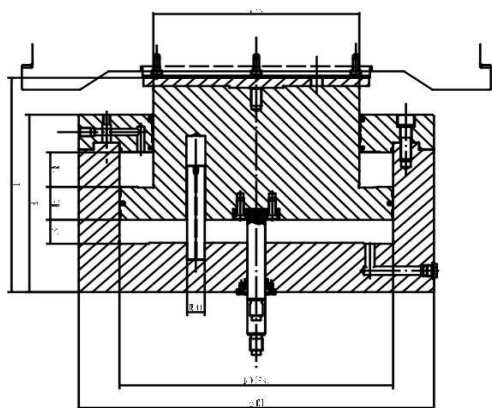
内置传感器内部防转结构
