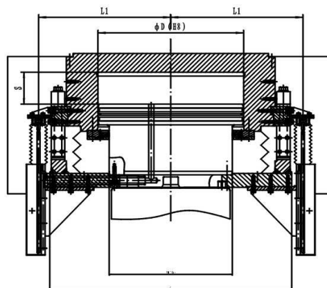
外置传感器外部防转结构
