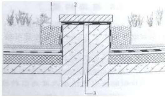
图 5.8.5 变形缝铺设盖板 1—卵石缓冲带；2—盖板；3—变形缝
