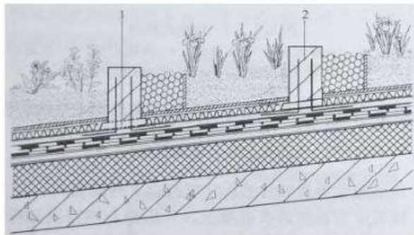
图 5. 3. 3-3 阶梯式种植 1—排水管(孔)；2—防滑挡墙
