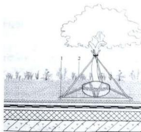
图 5.7.4-1 地上支撑固定法 1—稳固支架；2—支撑杆
