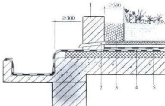
图 5. 5. 3 种植土挡墙构造
