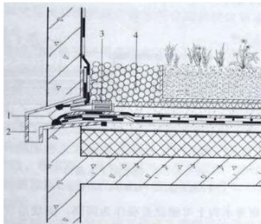
图 5.8.6 外排水 1—密封胶；2—水落口；3—雨算子；4—卵石缓冲带
