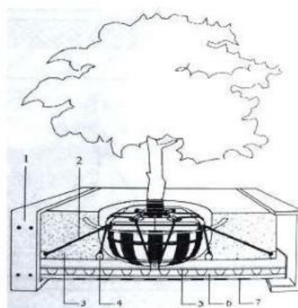
图 5.7.4-3 预埋索固法 1—种植池；2—绳索牵引；3—种植土；4—螺栓固定；5—过滤层；6—排(蓄)水层；7—耐根穿刺防水层
