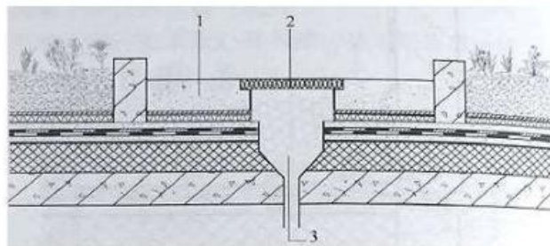
图 5.8.7-2 铺装层上水落口 1—铺装层；2—雨算子；3—水落口
