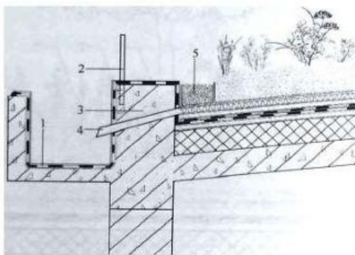
图 5.8.4 檐口构造 1—防水层；2—防护栏杆；3—挡墙；4—排水管；5—卵石缓冲带
