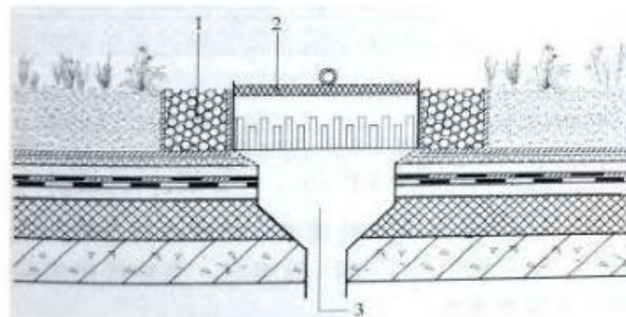
图 5.8.7-1 绿地内水落口 1—卵石缓冲带；2—井盖；3—雨水观察井
