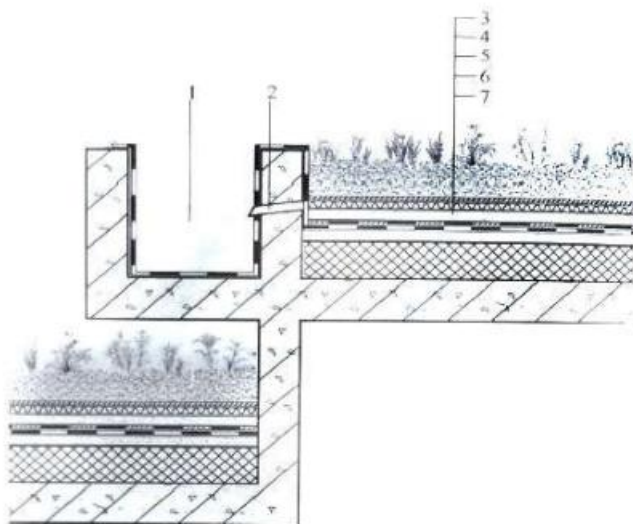
图 5.3.3-4 台地式种植
