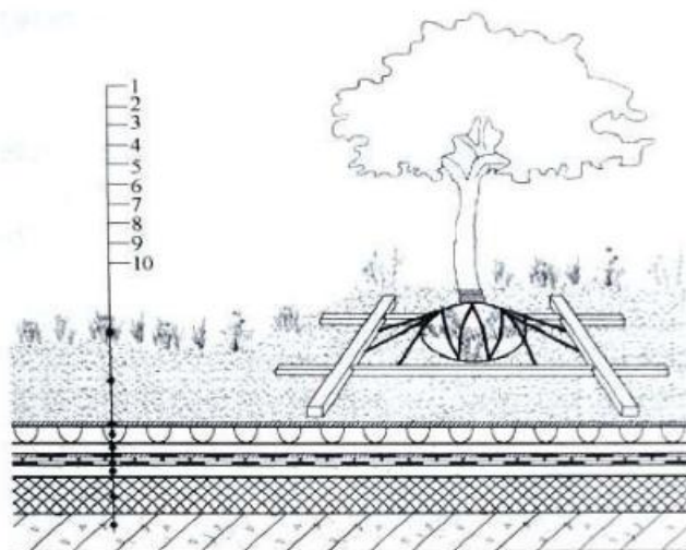
图 5.2.1 种植平屋面基本构造层次
