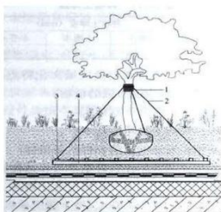
图 5.7.4-2 地上牵引固定法 1—软质衬垫；2—绳索牵引；3—螺栓铆固；4—固定网架
