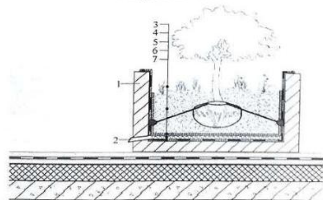
图 5.2.3 种植池
