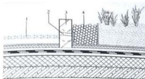
图2 硬质铺装排水
