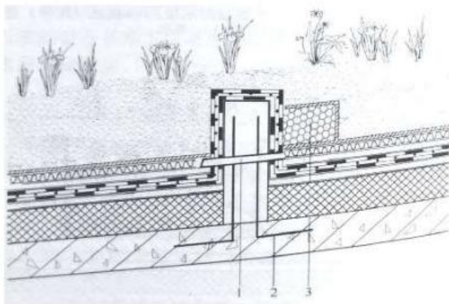
图 5. 3. 3-1 坡屋面防滑挡墙 1—排水管(孔)；2—预埋钢筋；3—卵石缓冲带
