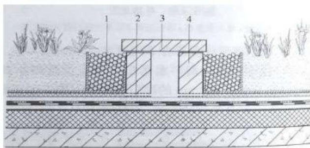
图 5.8.8 排水沟
