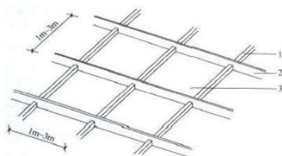
图 5. 3. 3-2 种植土防滑挡板 1—竖向支撑；2—横向挡板；3—种植土区域
