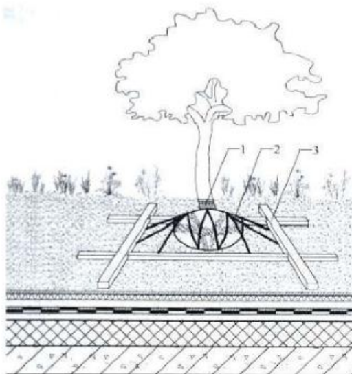
图 5.7.4-4 地下锚固法 1—软质衬垫；2—绳索牵引；3—固定支架
