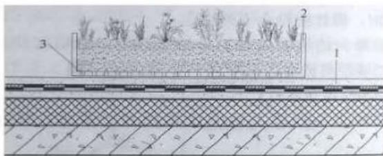
图 5. 6. 1 容器种植
