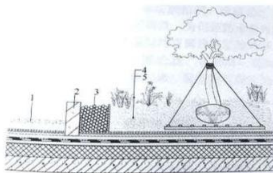
图3 植被层微地形处理
