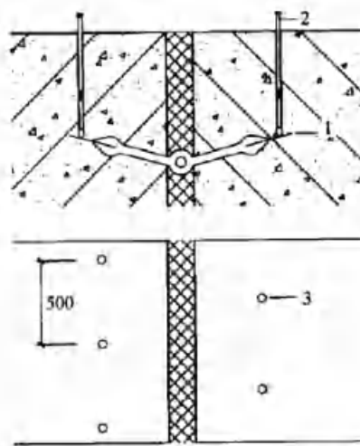
图 4.2.4-2 钻孔至止水带两翼 钢边并注浆止水
