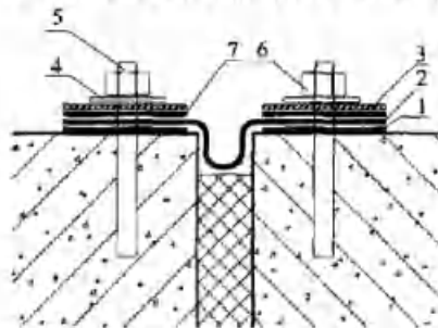
图 4.2.5-2 螺栓固定内置式密封止水带
