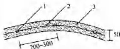
图 4.2.1-4 贴嘴注浆布孔 1—注浆嘴；2—裂缝；3—封缝材料
