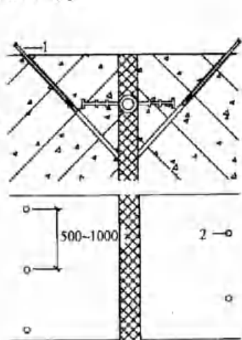
图 4.2.4-1 钻孔至止水带迎水面 注浆止水
