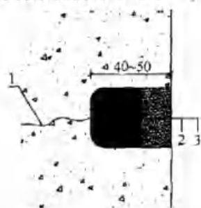
图 4.2.1-3 裂缝快速封堵止水 1—裂缝；2—速凝型无机防水堵漏材料； 3—聚合物水泥防水砂浆
