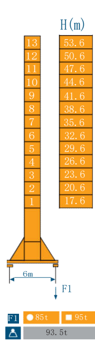
行走式 Travelling
