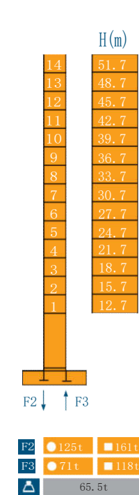
固定式 Stationary
