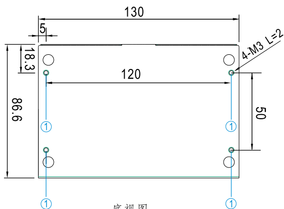
底视图
