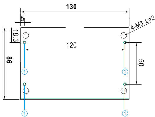
底视图
