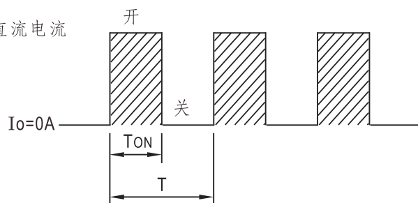
◎PWM形式输出
