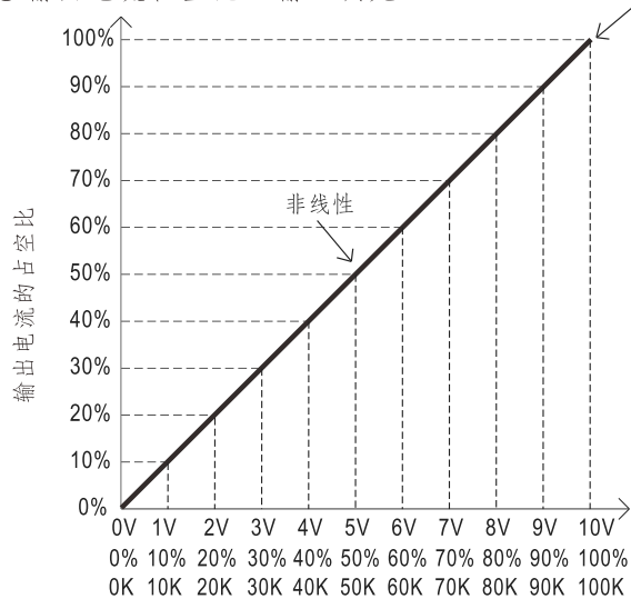
◎输出电流占空比VS输入调光
