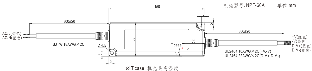
■ 机构尺寸
