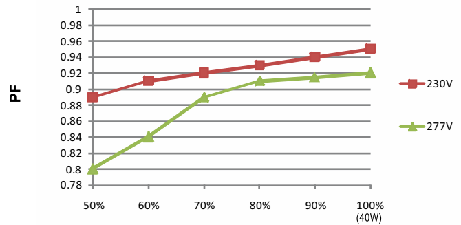
负载 E 型
