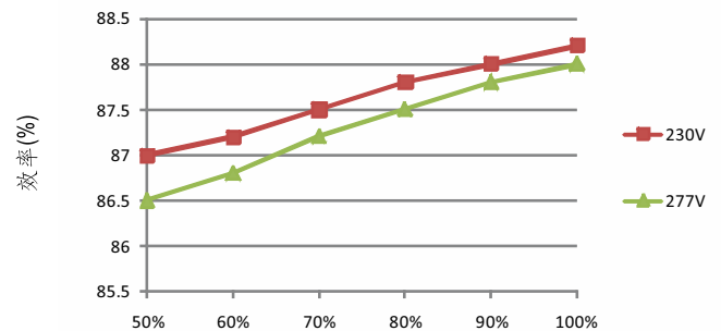
负载 E 型
