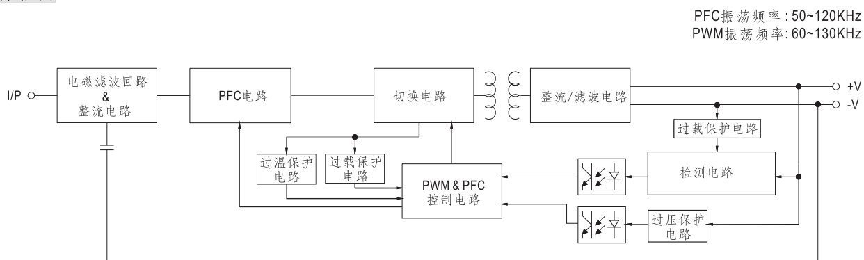
■ 方框图
