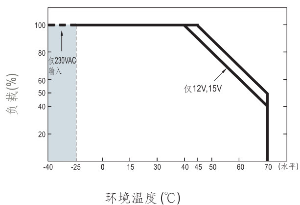
■ 减额曲线
