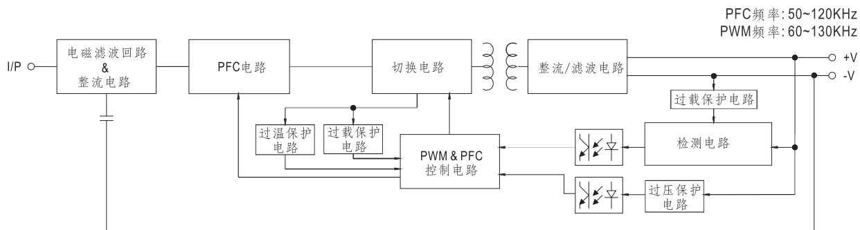
■ 方框图
