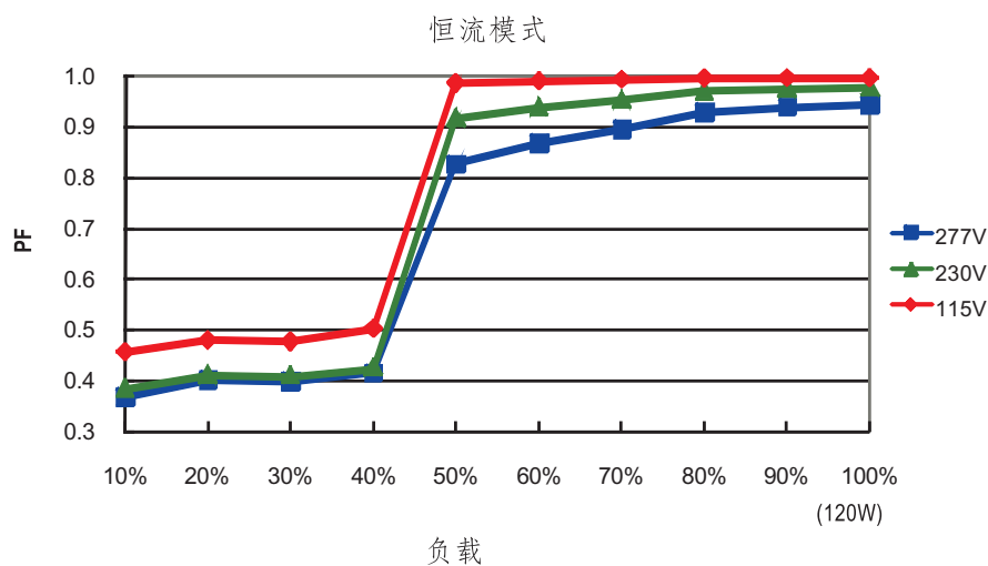
■ 功率因素特性
