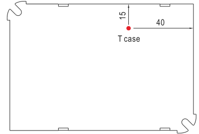
底视图
