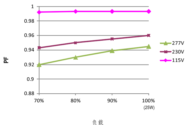
■ 功率因素特性曲线
