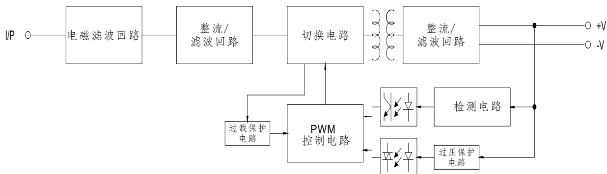
■ 方框图
