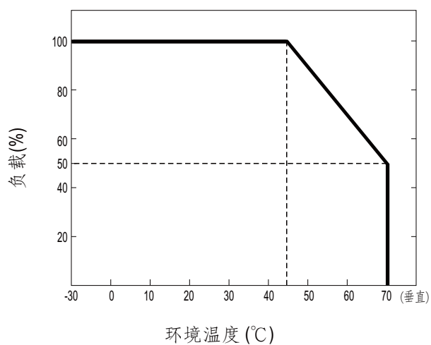
■ 减额曲线
