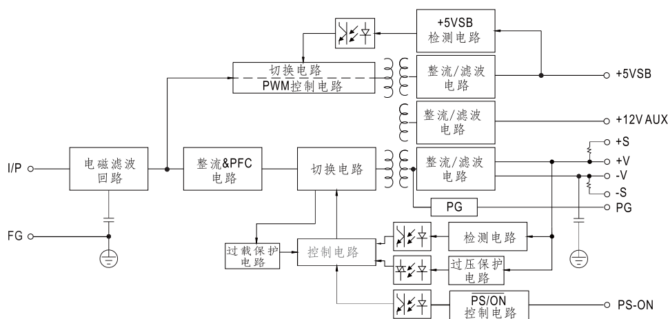
■ 方框图
