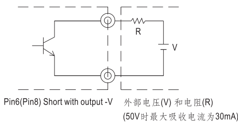
图2.2 AC OK内部电路(电池低压),采用TTL集电极开路
