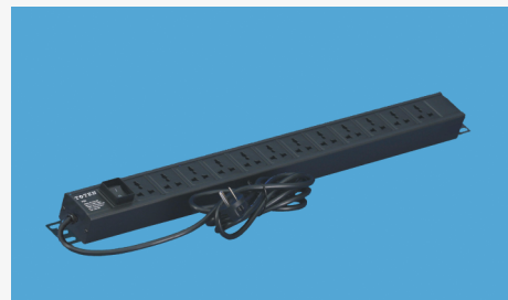
12位国标PDU, 10A输入输出，带总开关， 线长3M，反方向安装，带TOTEN丝印 (PD.1201.9000)
