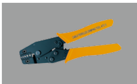
■ 1530 歐式端子壓著鉗 ■ CABLE FERRULES CRIMPING TOOL KTC-5 適用端子: 0.5-0.75 mm 2 /1.0-1.5 mm 2 /2.5 mm 2 /4 mm 2 6 mm 2
