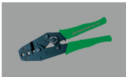
■ 1530 歐式端子壓著鉗 ■ CABLE FERRULES CRIMPING TOOL KTC-17 適用端子: 25 mm 2 /35 mm 2
