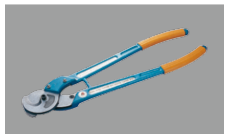
■ 1530 電纜剪 ■ CABLE CUTTERS RYC-60 適用電纜:最大60sq / AWG 1/0 / DIN 50mm 2 RYC-100 適用電纜:最大100sq / AWG 4/0 / DIN 120mm 2 RYC-250 適用電纜:最大250sq / AWG 500mcm / DIN 260mm 2 RYC-400 適用電纜:最大400sq / AWG 600mcm / DIN 300mm 2 RYC-500 適用電纜:最大500sq
