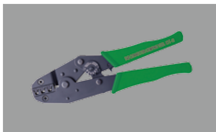
■ 1530 強力壓著不絕緣端子鉗 ■ TAB CONNECTOR CRIMPING TOOL KTT-12 適用裸端子: 1.1-2.5 mm 2 /4-6 mm 2 /6-8 mm 2
