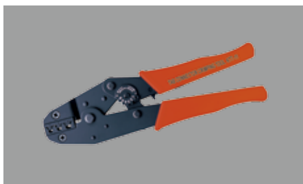
■ 1530 強力壓著不絕緣端子鉗 ■ TAB CONNECTOR CRIMPING TOOL KTT-11 適用裸端子: 0.5-10 mm 2 /1.1-2.5 mm 2 /4-6 mm 2
