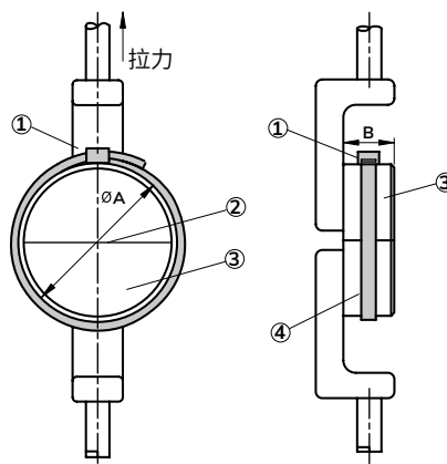
圖2.平行穿入式紮線帶頭部需在上方
