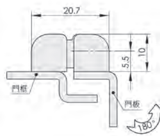
CL-203-4L(左/L) CL-203-5R(右/R) 小型偏置鉸鏈
