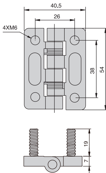
CL-209-1R 螺柱型 Thread-stud Type
