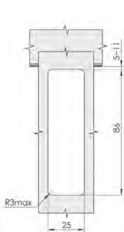
開孔尺寸 Cut Out
