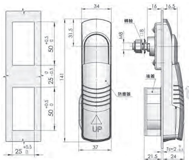
開孔尺寸 Cut Out
