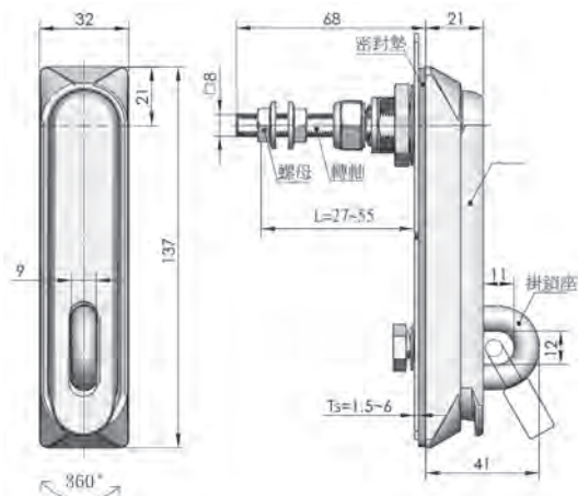
掛鎖示意圖
