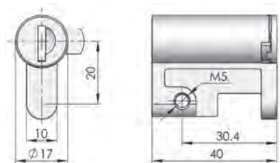
標準鎖芯 Standard Lock Cylinder
