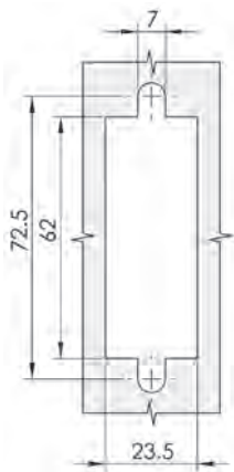
開孔尺寸 Cut Out
