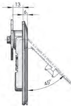
MS-723-3 (無鎖芯 Non Locking)
