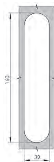
開孔尺寸 Cut Out
