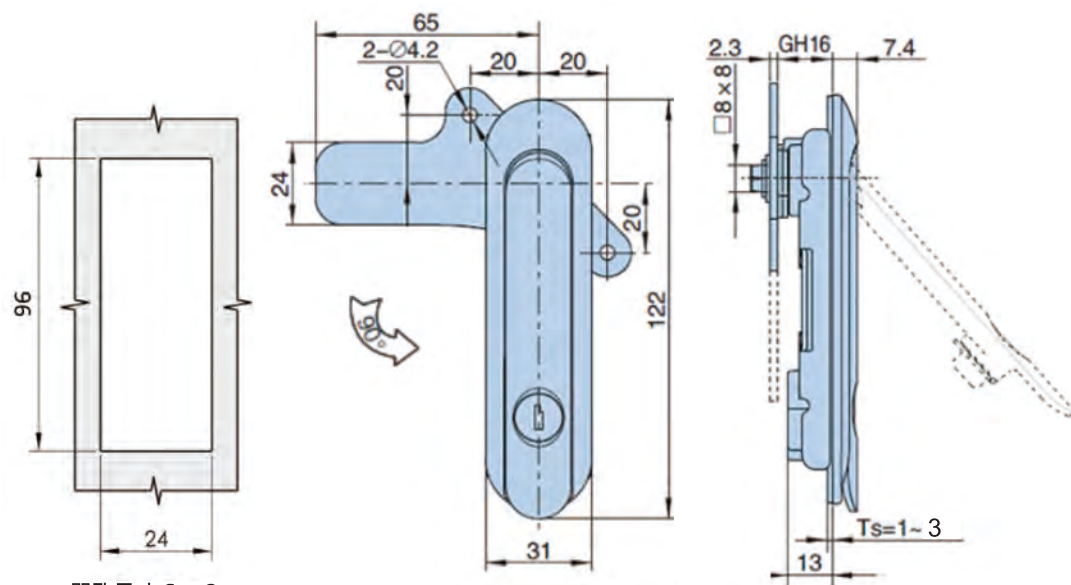
開孔尺寸 Cut Out
