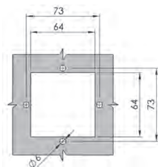
開孔尺寸 Cut Out
