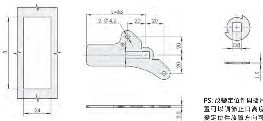
開孔尺寸 Cut Out
