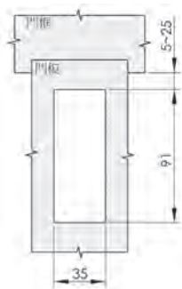
開孔尺寸 Cut Out
