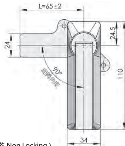
MS-723-3 (無鎖芯 Non Locking)
