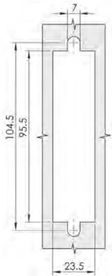
開孔尺寸 Cut Out
