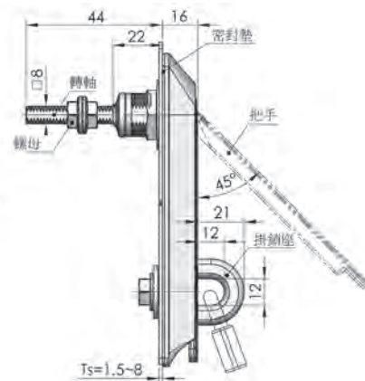
掛鎖示意圖
