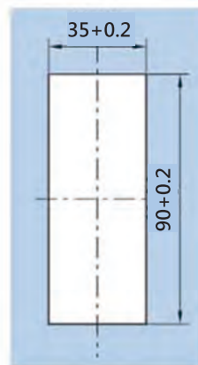
開孔尺寸 Cut Out
