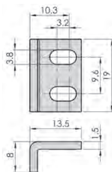
固定扣
