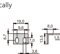
固定扣
