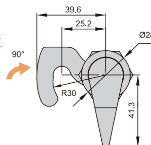
標準擋片
