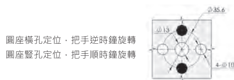
開孔尺寸 Cut Out
