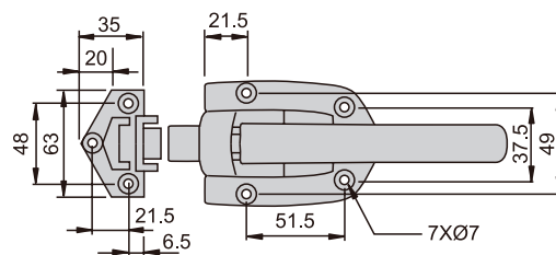
AH-52-A 高扣座
