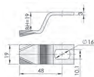
擋片
