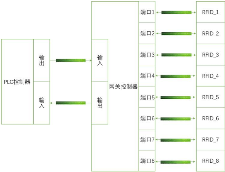
图 6-1 通讯架构图
