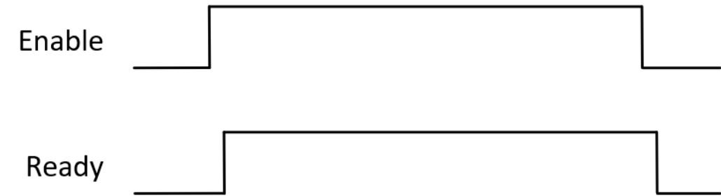
图 6-2 RFID 使能时序图
