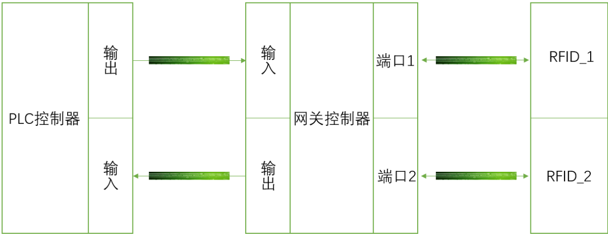
图 6-1 通讯架构图
