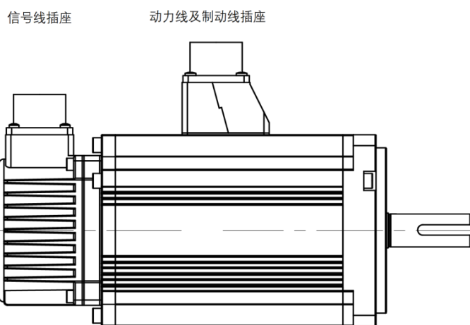
图 1.3.2-2 电机铭部件名称
