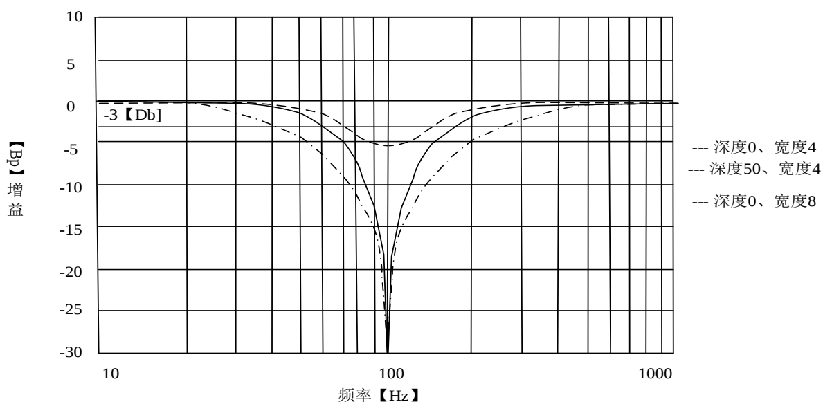
图 7.2.6-1 陷波滤波器频率特性
