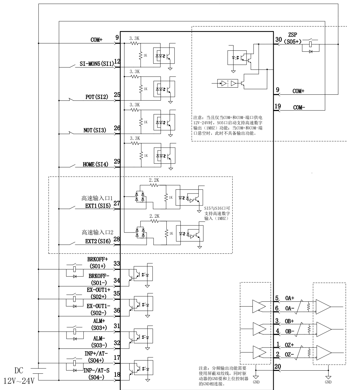
图 2.9-1 连接器 CN1 输入输出 NPN 型接法
