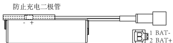
图 9.5.1-2 电池盒接线定义图
