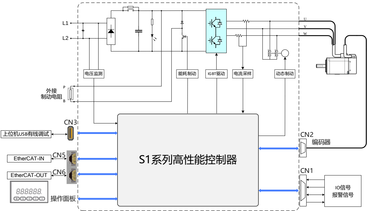
图 1.2.4-1 系统框图
