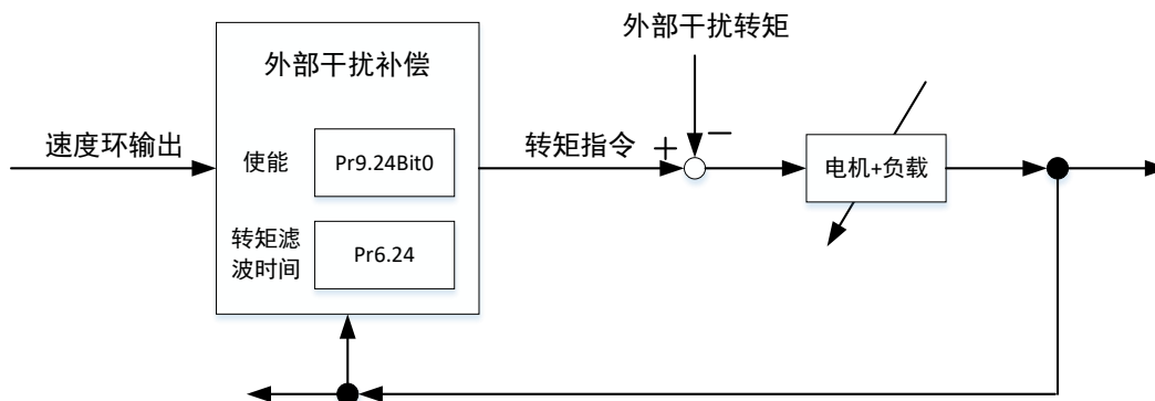
7.2.9- 1 负载变动抑制功能
