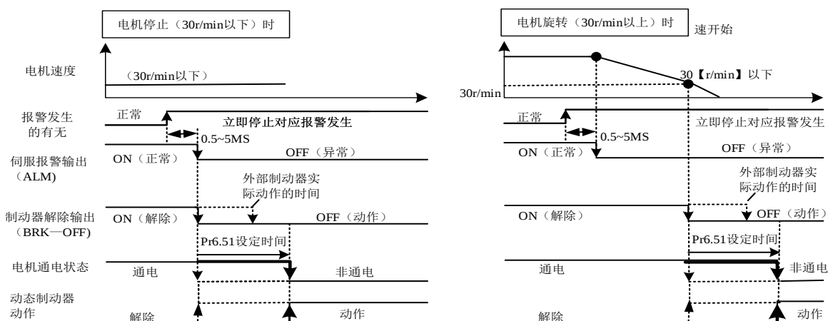
图 10.2.6-1 报警发生时的立即停止动作
