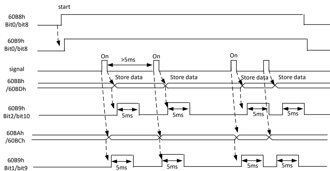
图 10.8-7 连续上升沿下降沿触发
