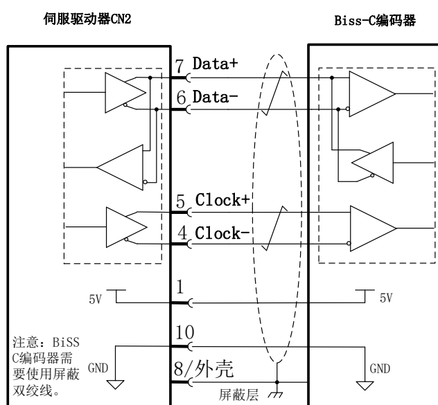
图 2.3.2-5 BiSS C 编码器接线
