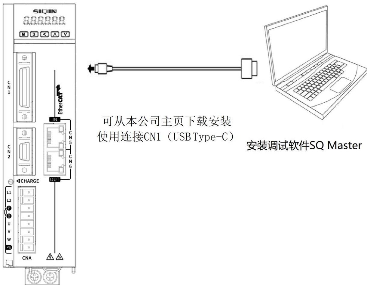
图 3.2.1-1 驱动器与 PC 连接方式
