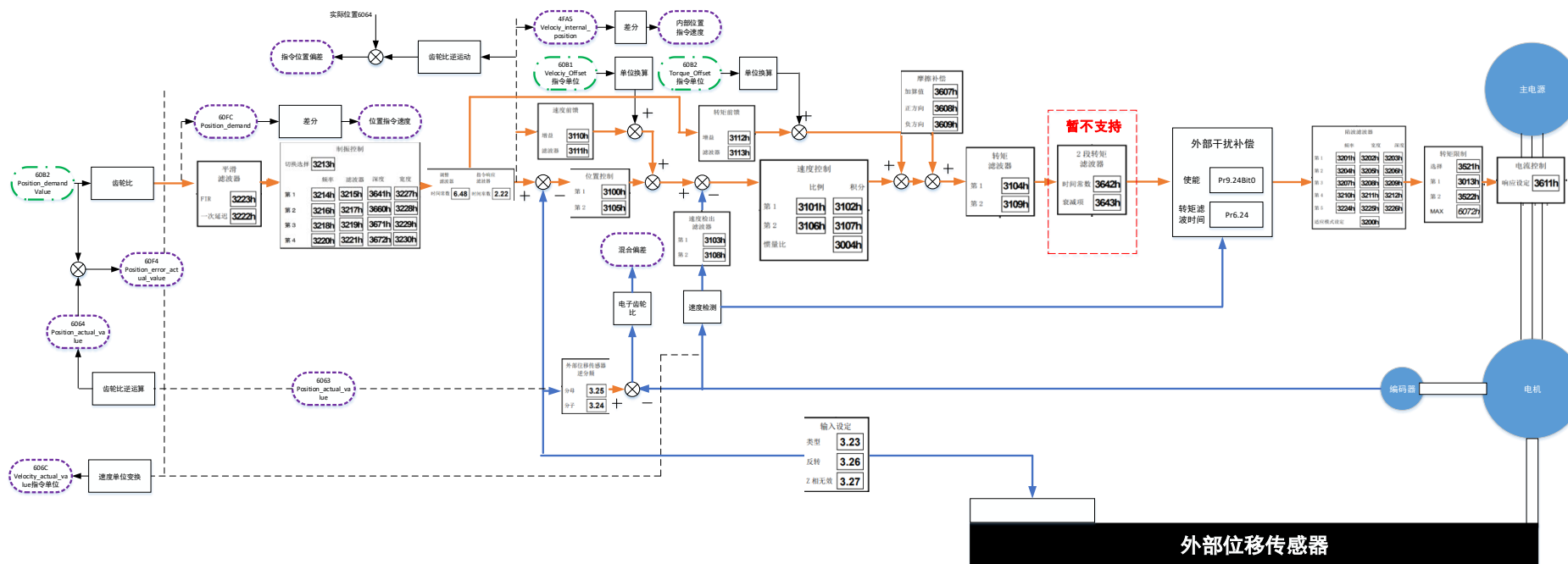
图 7.2.16-1 2 自由度控制模式（全闭环控制）Block
