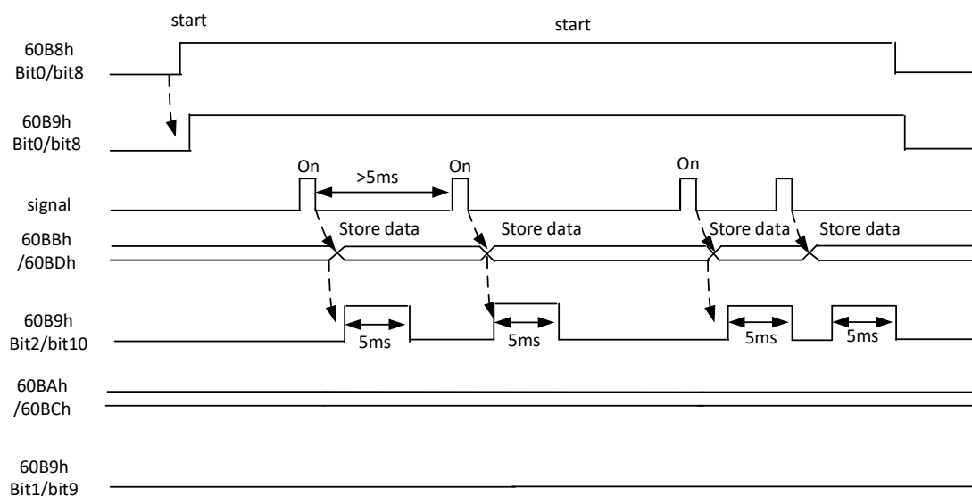
图 10.8-6 连续下降沿触发
