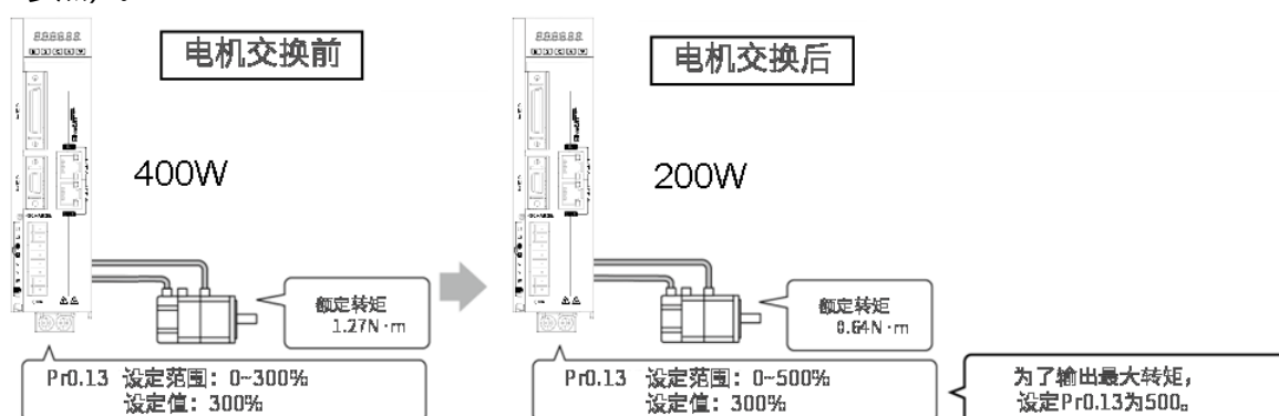
图 3.2.4-1 电机最大转矩输出时
