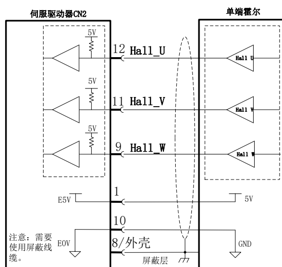
图 2.3.2-4 单端霍尔编码器接线
