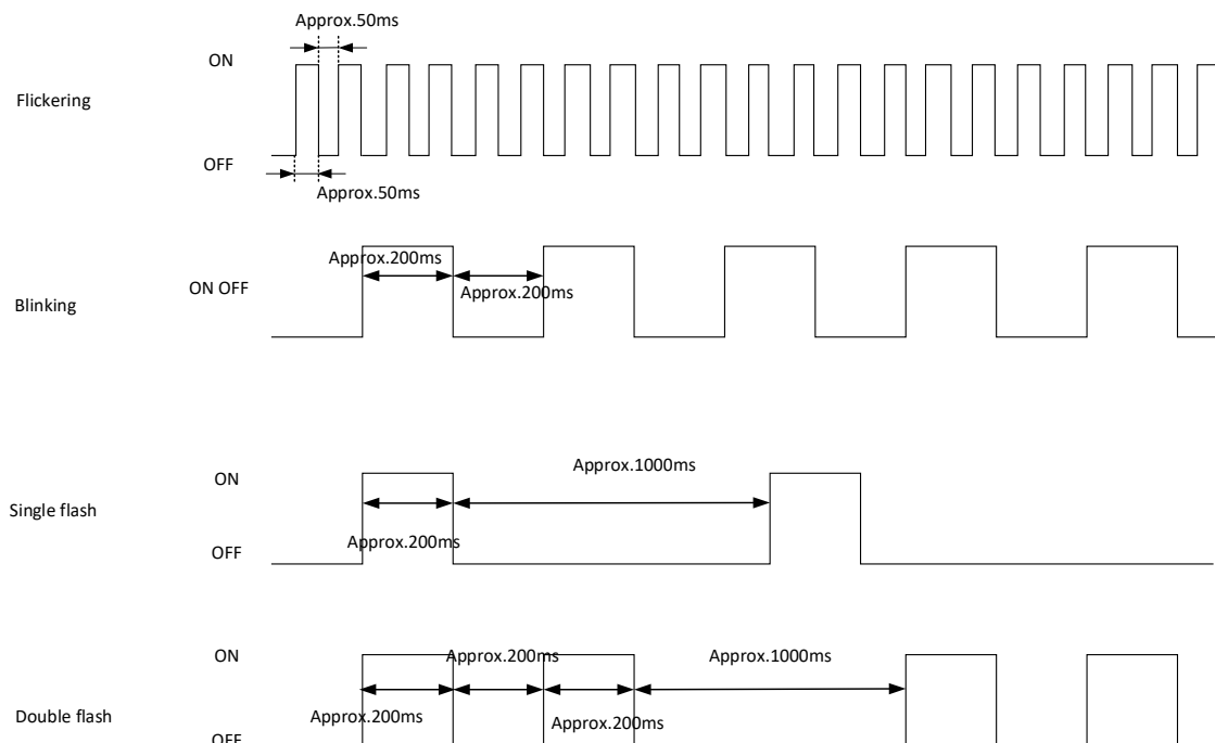
图2.7.3-1 EtherCAT 指示灯 4种模式
