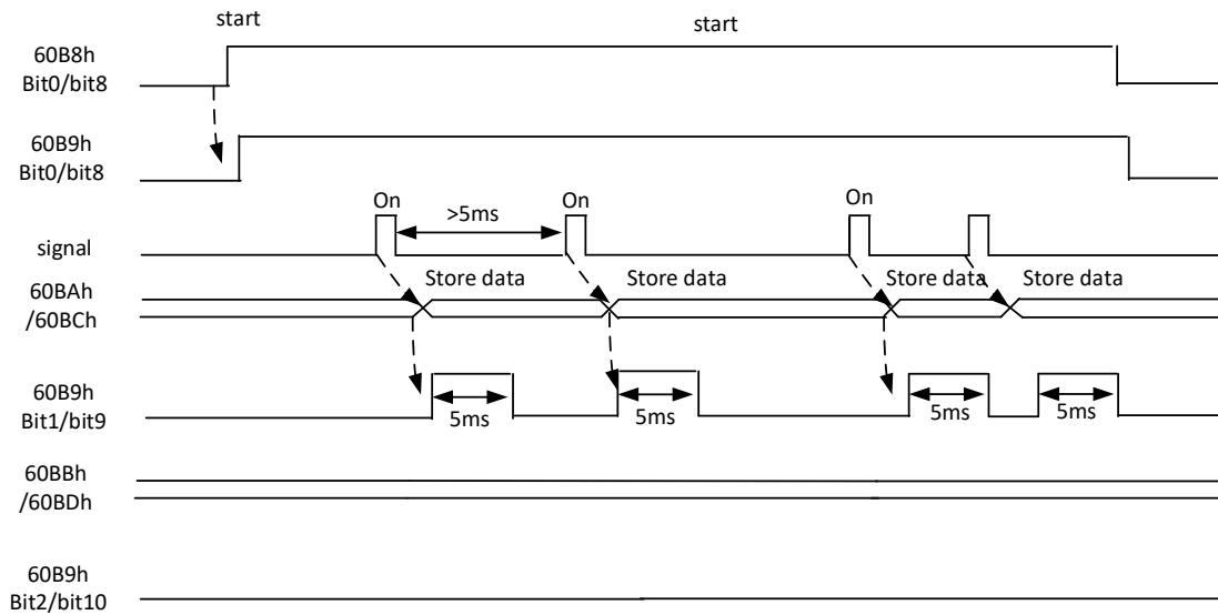
图 10.8-5 连续上升沿触发
