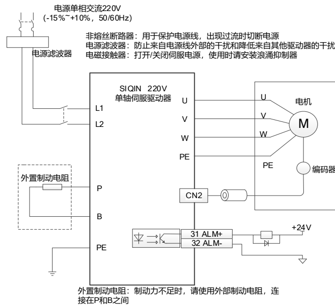
图 2.2.1-1 单相 220V 配线图
