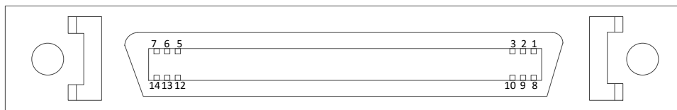
图 2.3.2-1 CN2 接口
