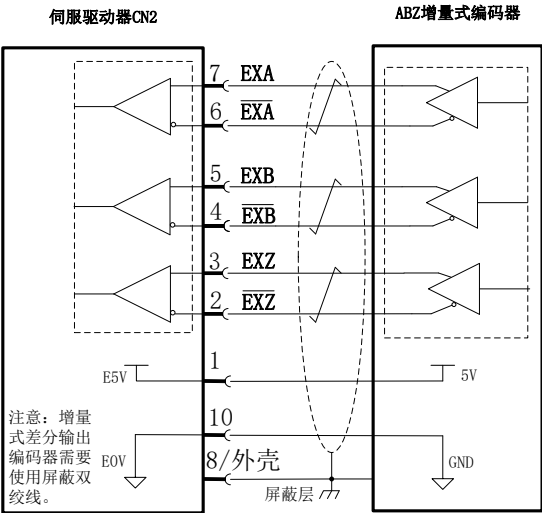
图 2.3.2-3 ABZ 增量式编码器接线
