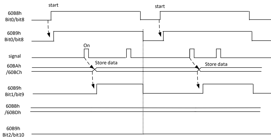
图 10.8-2 单次上升沿触发
