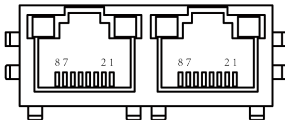
图 2.3.4-1 CN5/CN6 接口
