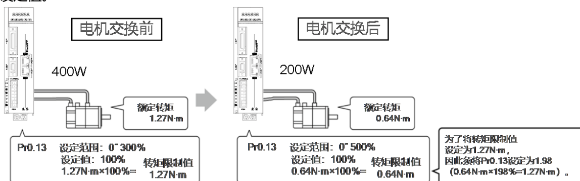
图 3.2.4-1 限制电机的转矩时
