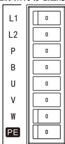
图 2.3.5-1 CNA 接口
