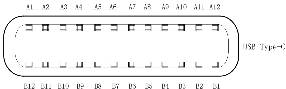
图 2.3.3-1 CN3 接口
