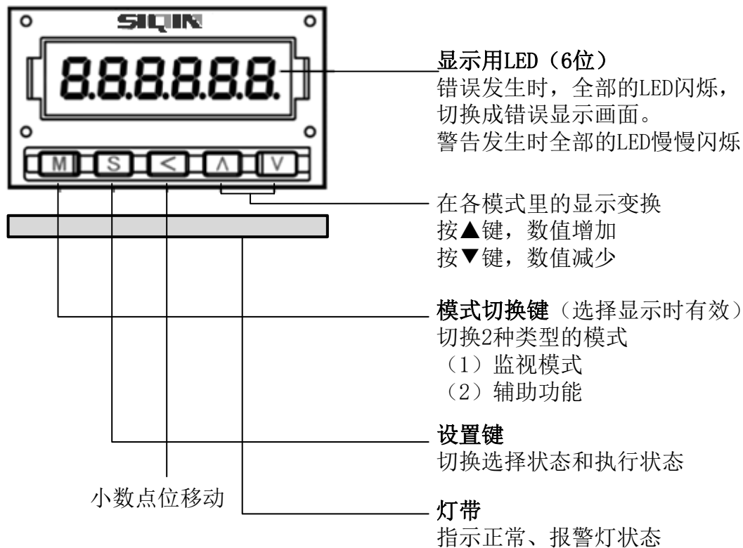
图 2.7.1-1 前面板构成
