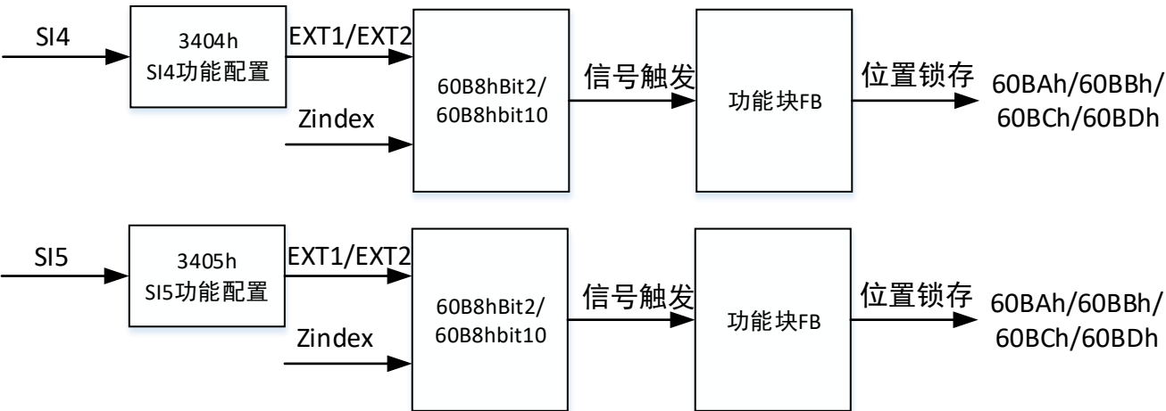
图 10.8-7 探针功能描述
