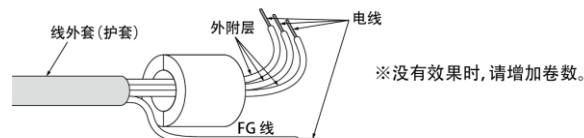
图 2.1-3 磁环连接图
