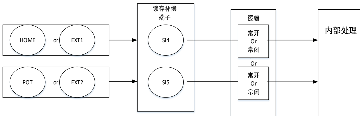
图 2.10.4-1 输入输出信号的分配
