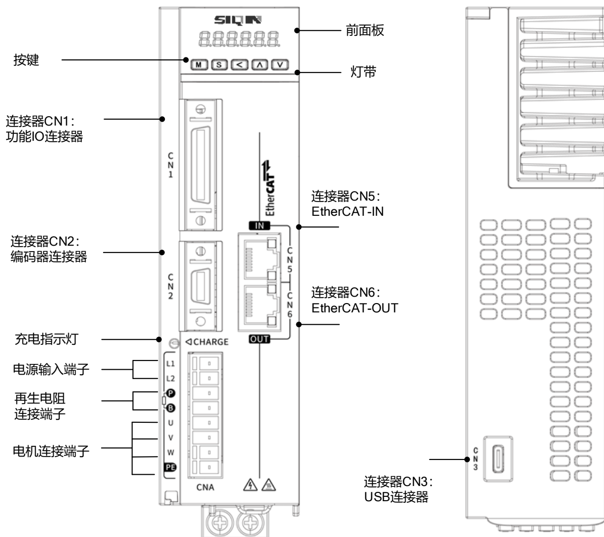
图 1.2.2-1 驱动器各部分名称
