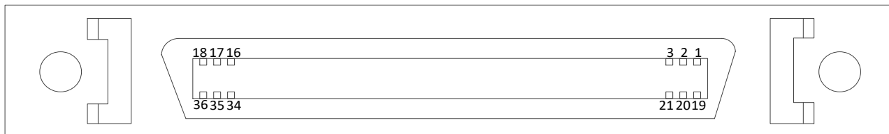
图 2.3.2-1 CN1 接口
