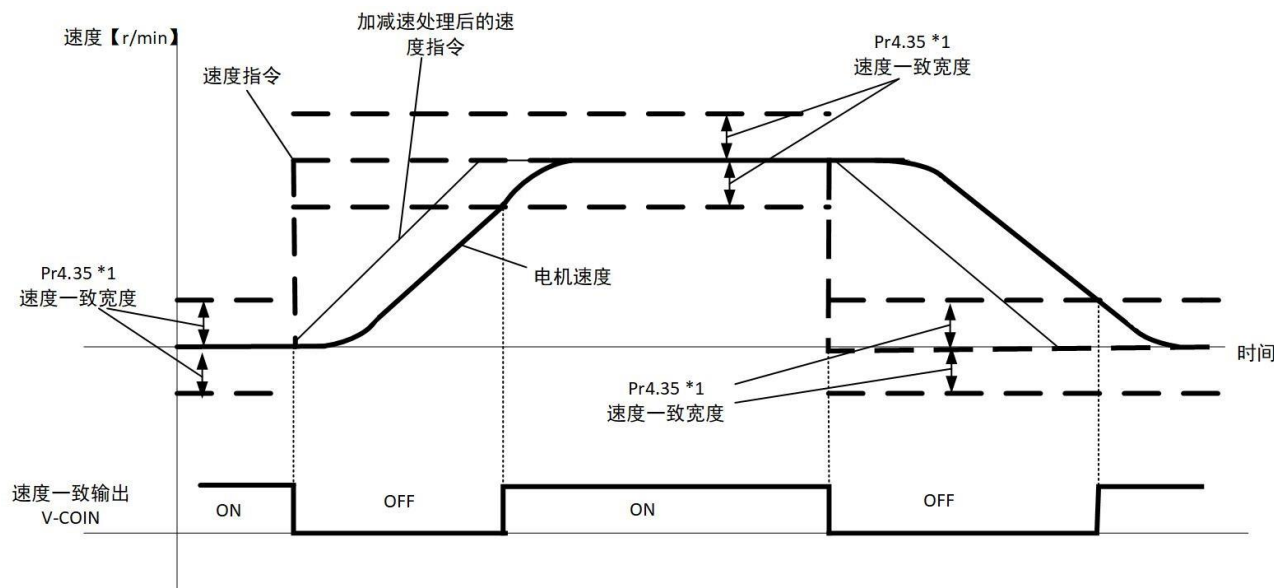
图5.3.2-1 速度指令与速度一致时的波形
