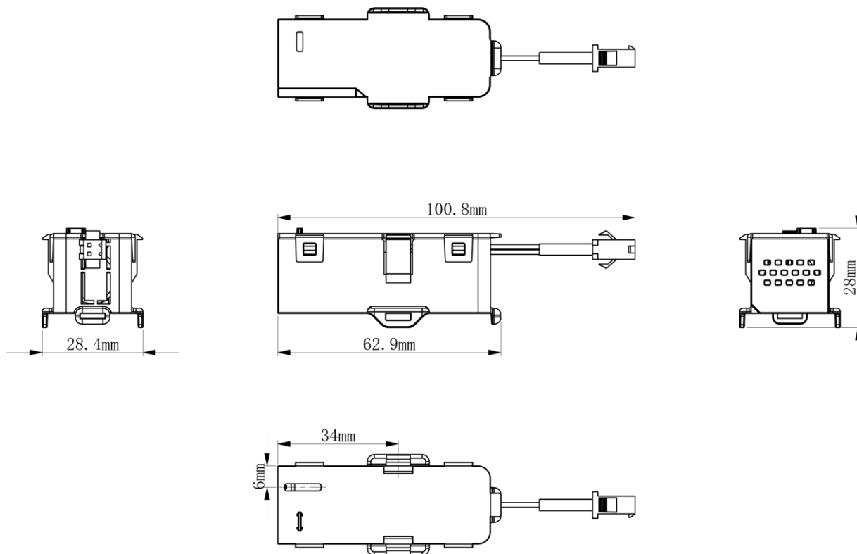
图 9.5.1-1 电池盒外形尺寸图
