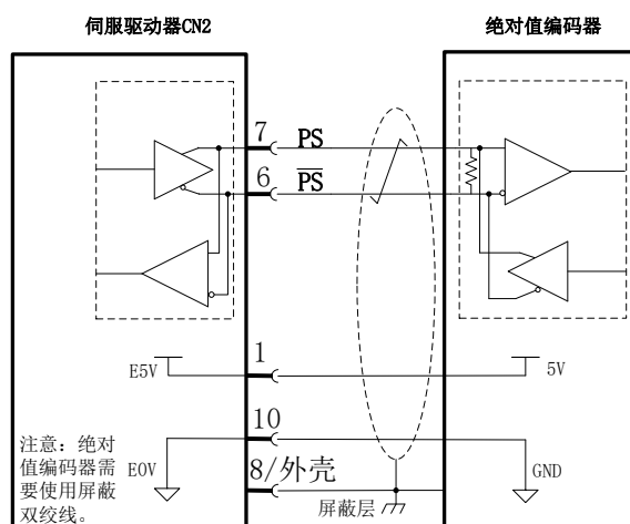
图 2.3.2-2 绝对值编码器接线
