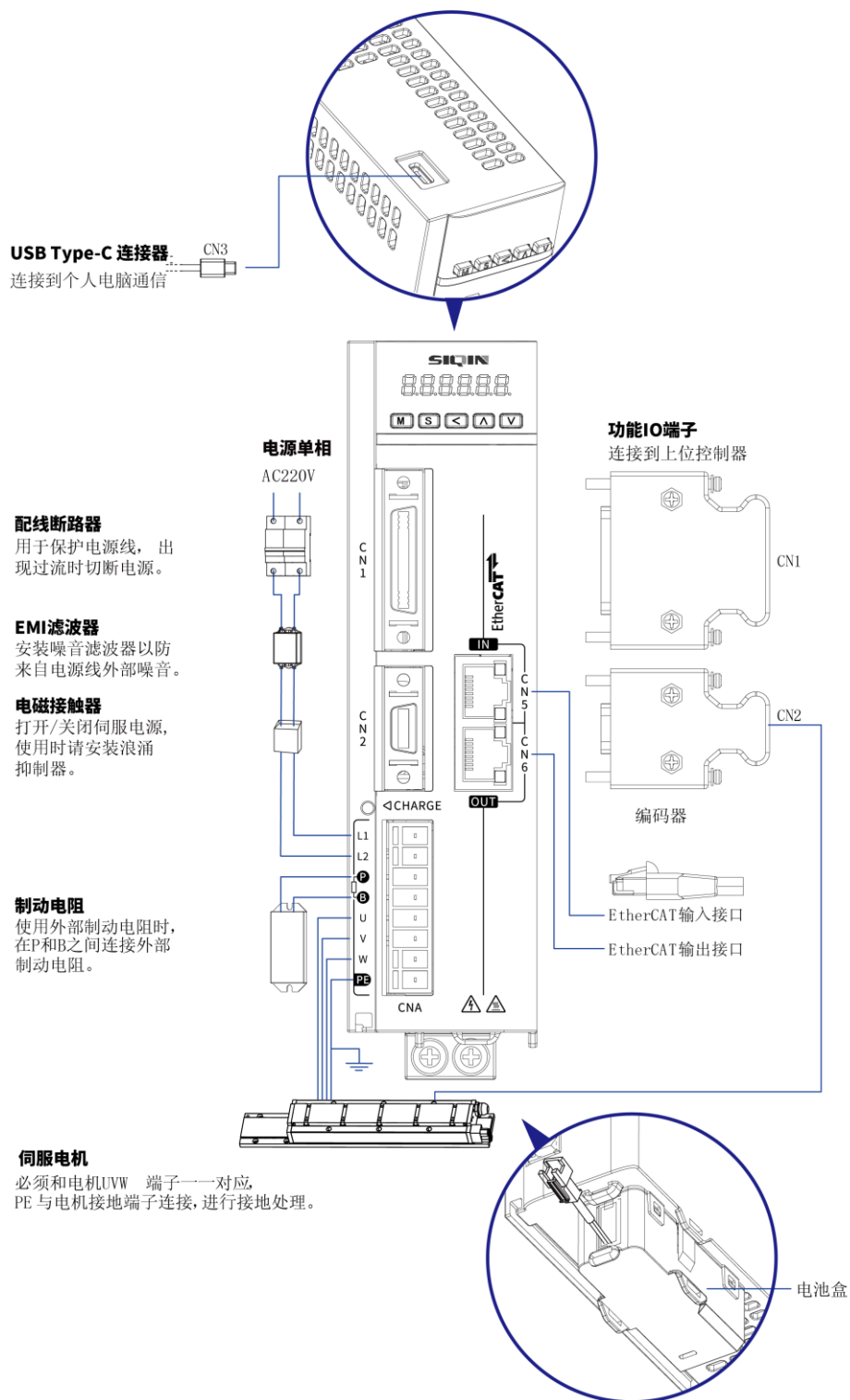
图 2.2.2-1 A 型驱动器配线图
