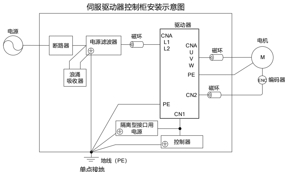
图 2.1-1 控制箱图
