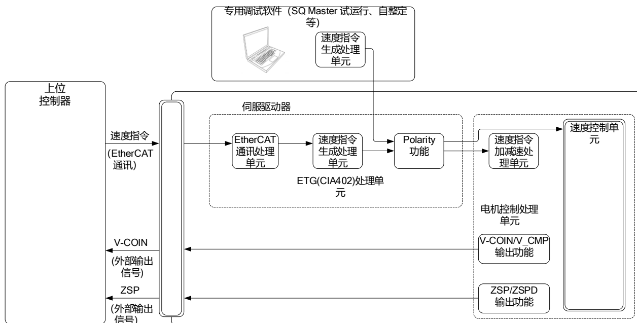
图 5.3-1 速度控制的设定
