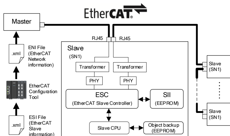
图 4.2-1 EtherCAT 主站 从站构成图
