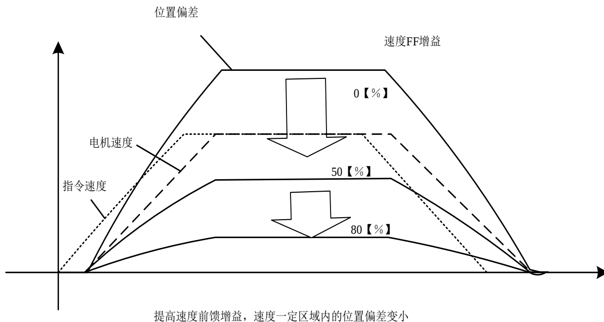
图 7.2.8-1 速度前馈功能
