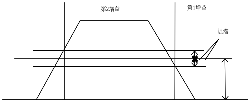
图 7.2.5-2 切换等级与迟滞的设定
