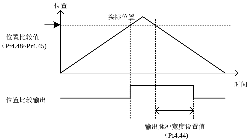
图 10.4-2 动作方向反转时且设定多个位置比较值时的位置比较输出
