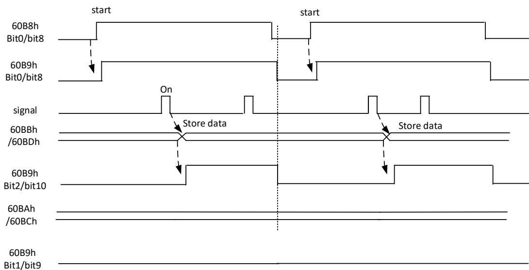
图 10.8-3 单次下降沿触发
