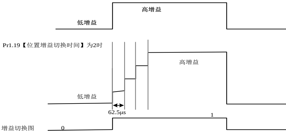
图 7.2.5-4 位置增益切换时间的设定
