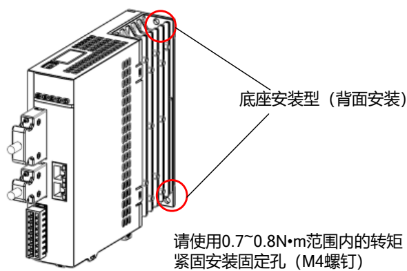
图 1.5.1-1 驱动器安装孔位置
