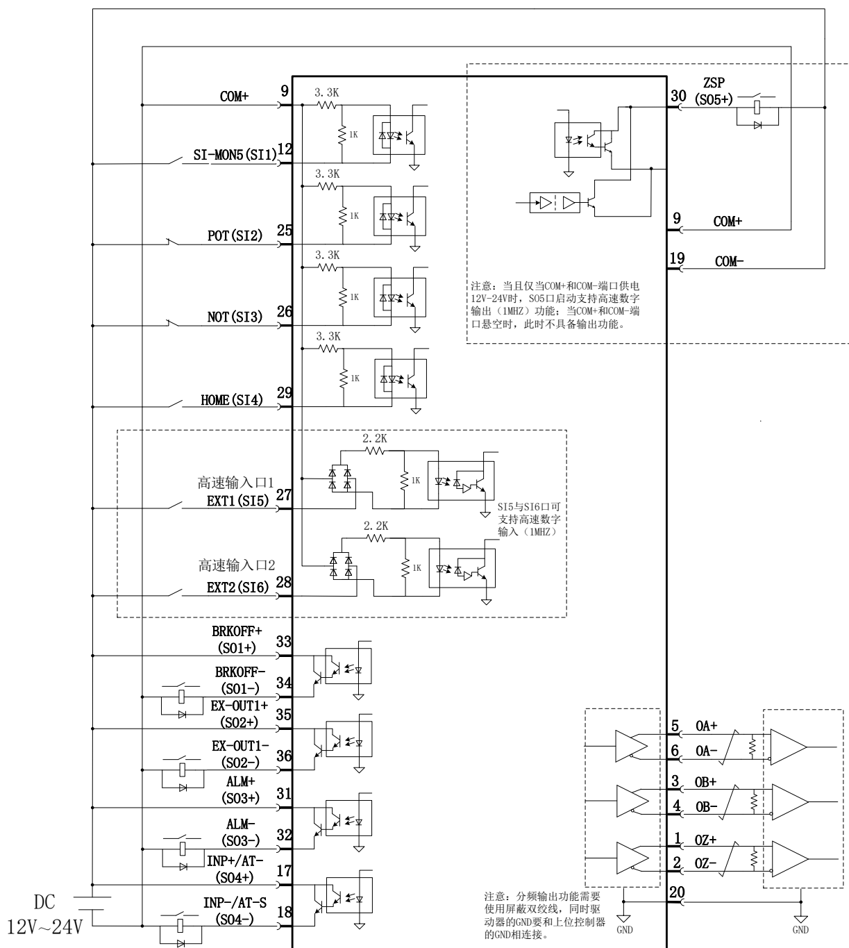
图 2.9-2 连接器 CN1 输入输出 PNP 型接法
