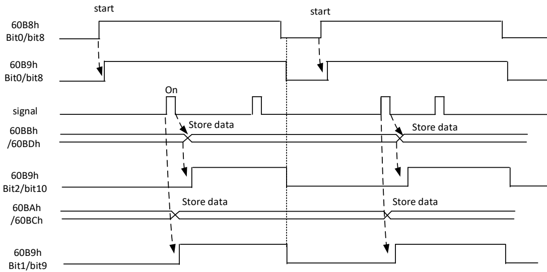
图 10.8-4 单次上升沿下降沿触发
