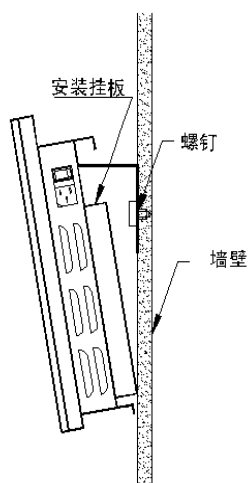
图2：挂墙安装示意图
