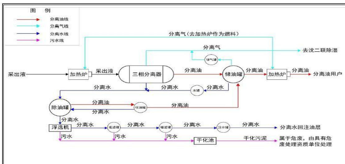
图 1-4 生产工艺流程图
