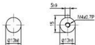
轴型式 S1
