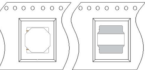
产品摆放方向顶视图
