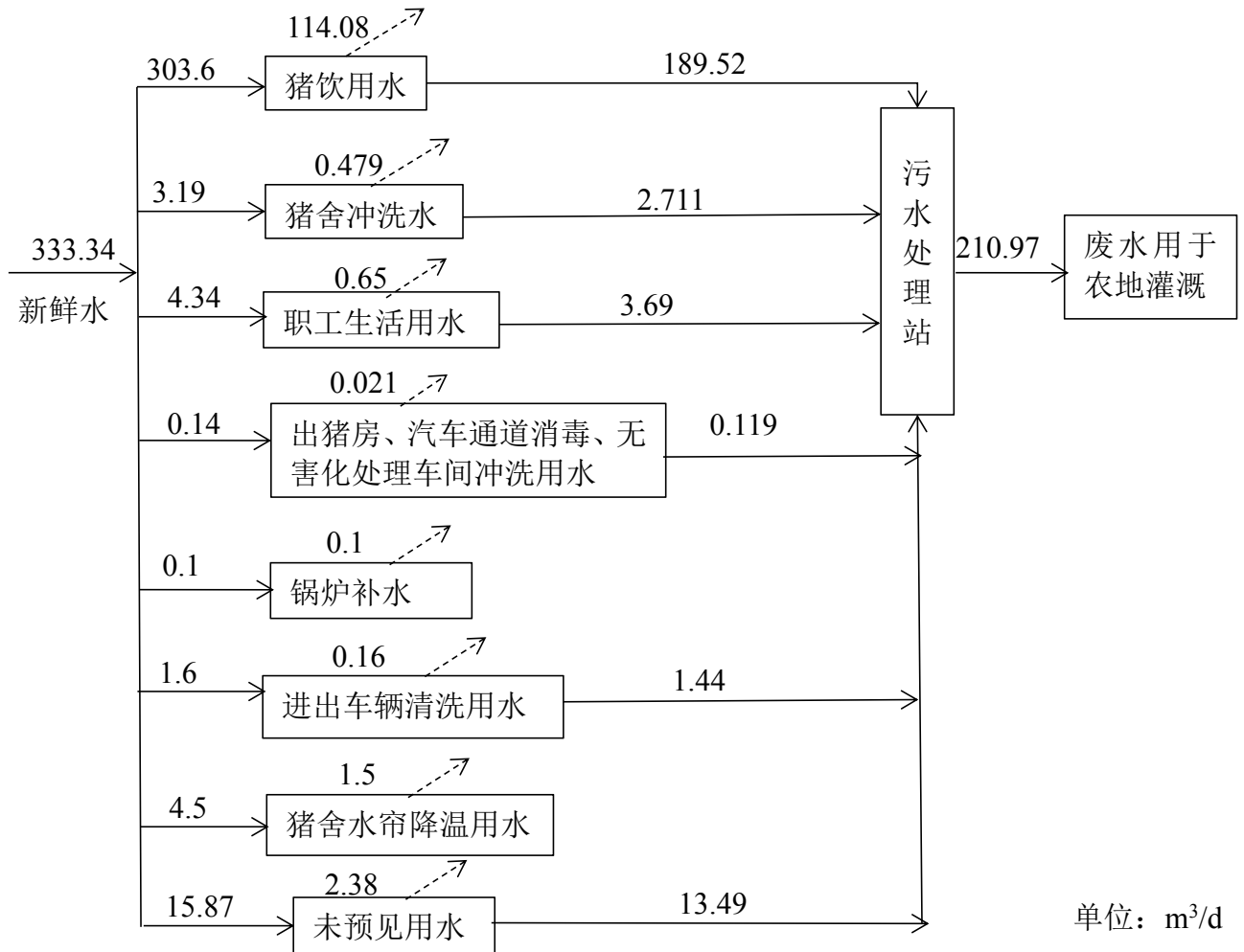
图 2.2-6 项目水平衡图
