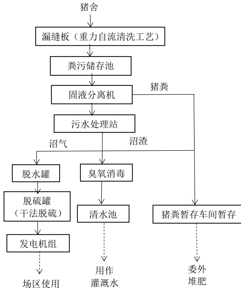
图 2.2-2 粪污处理及综合利用工艺图
