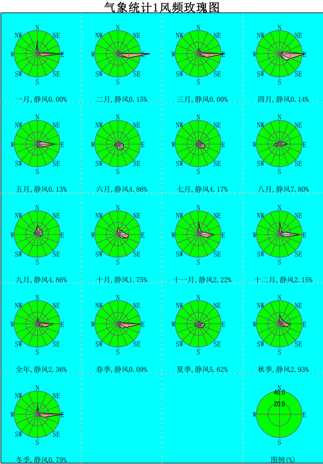
图 5.2-7 湛江市 2019 年地面风向玫瑰图
