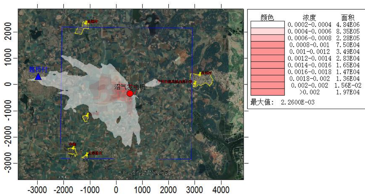
图 5.2-13 NO 2 日平均浓度预测值分布图
