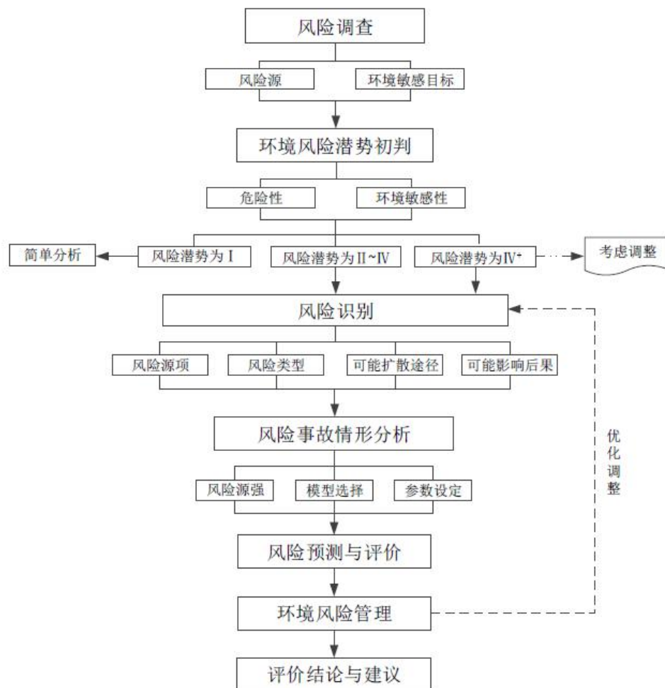
图 5.2-24 环境风险评价工作程序
