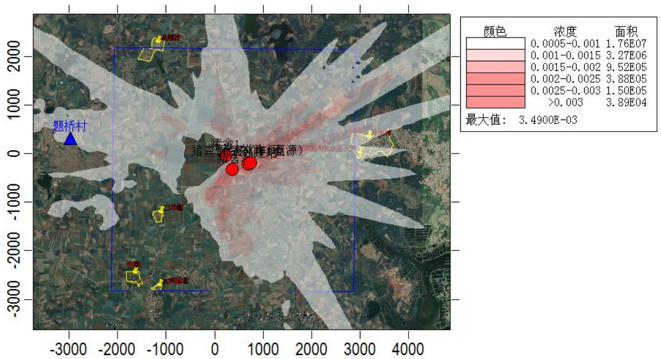
图 5.2-18 H 2 S 小时浓度预测值分布图
