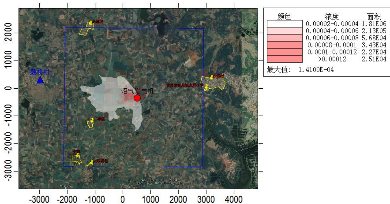
图 5.2-10 \text{SO}_2 日平均浓度预测值分布图
