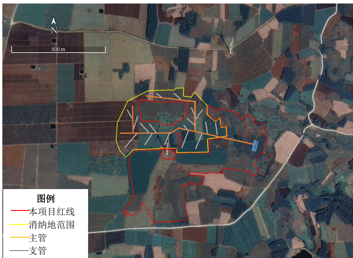
图 5.2-22 废水管道灌溉农地示意图
