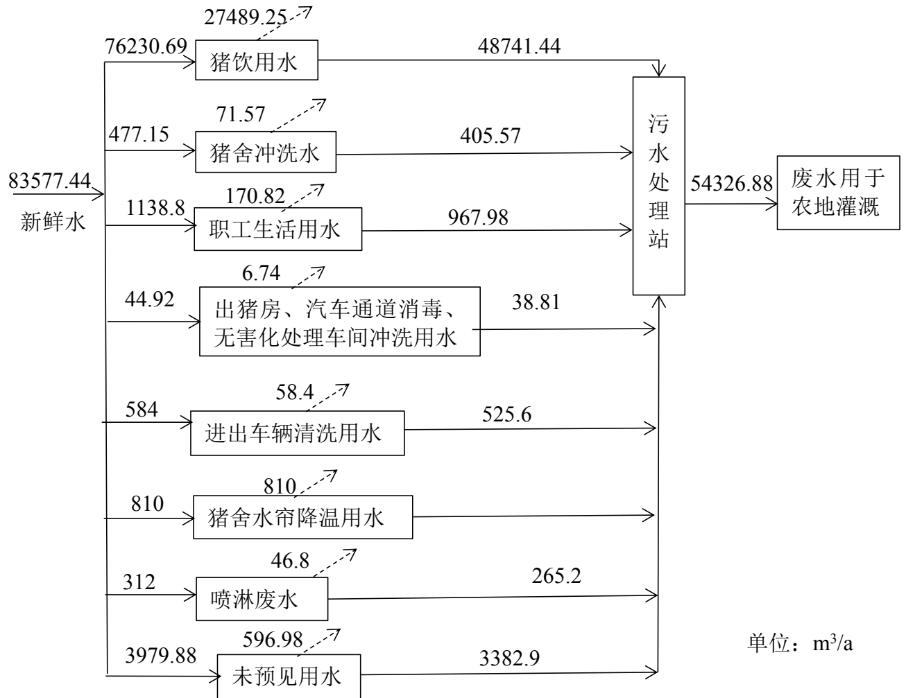
图 2.2-6 项目水平衡图
