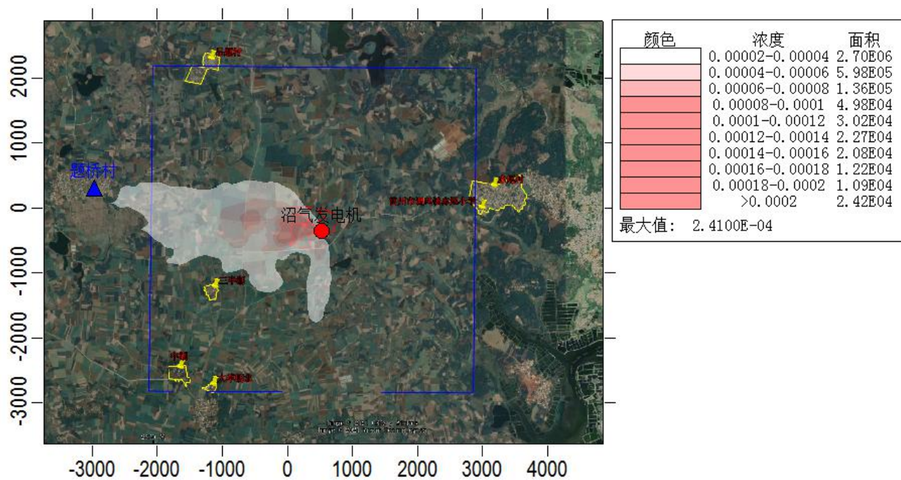
图 5.2-16 PM 10 年平均浓度预测值分布图
