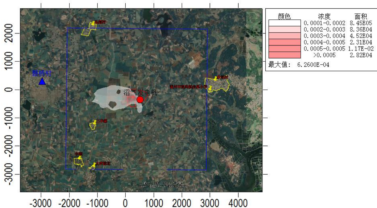
图 5.2-14 NO 2 年平均浓度预测值分布图
