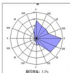
图 5.2-3 湛江市近 20 年风向玫瑰图
