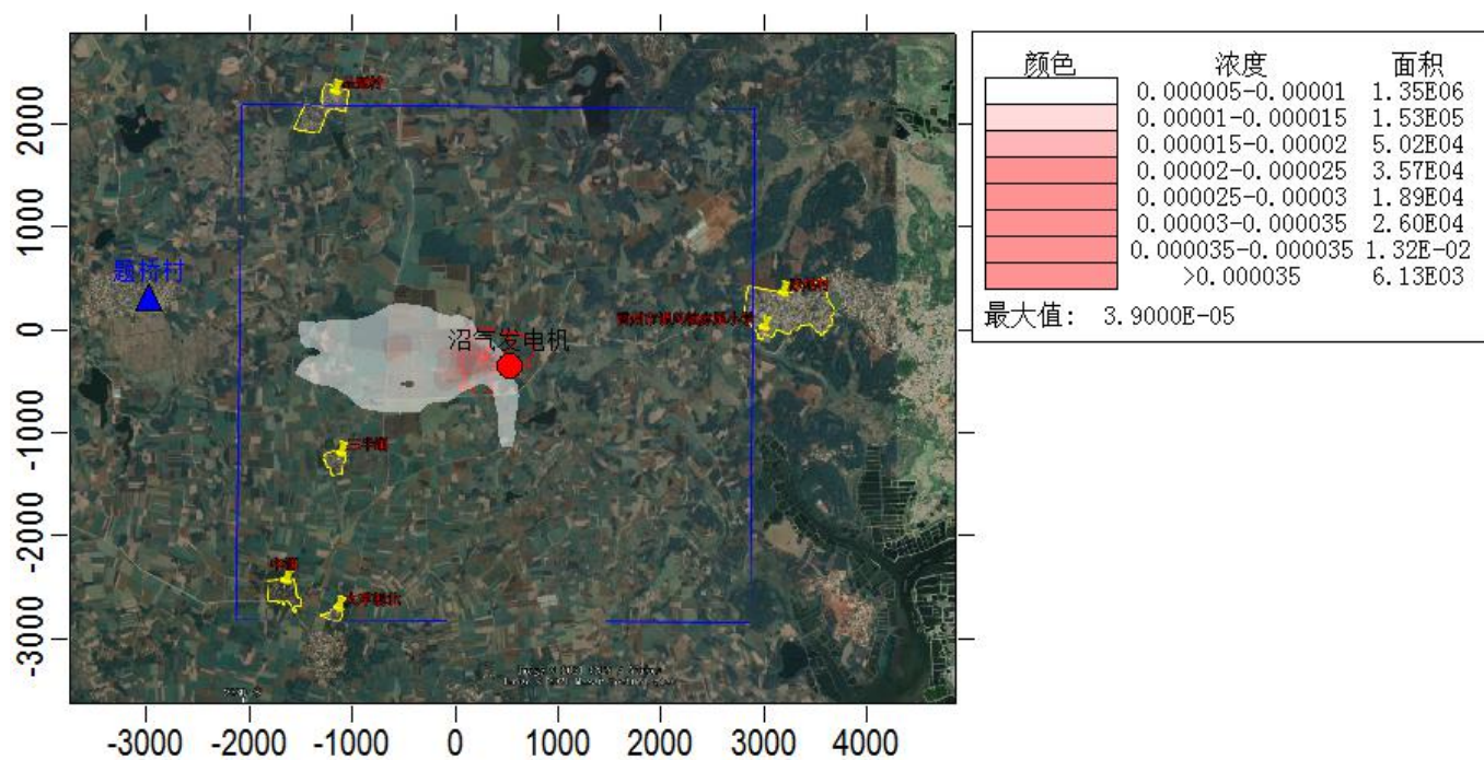
图 5.2-11 \text{SO}_2 年平均浓度预测值分布图
