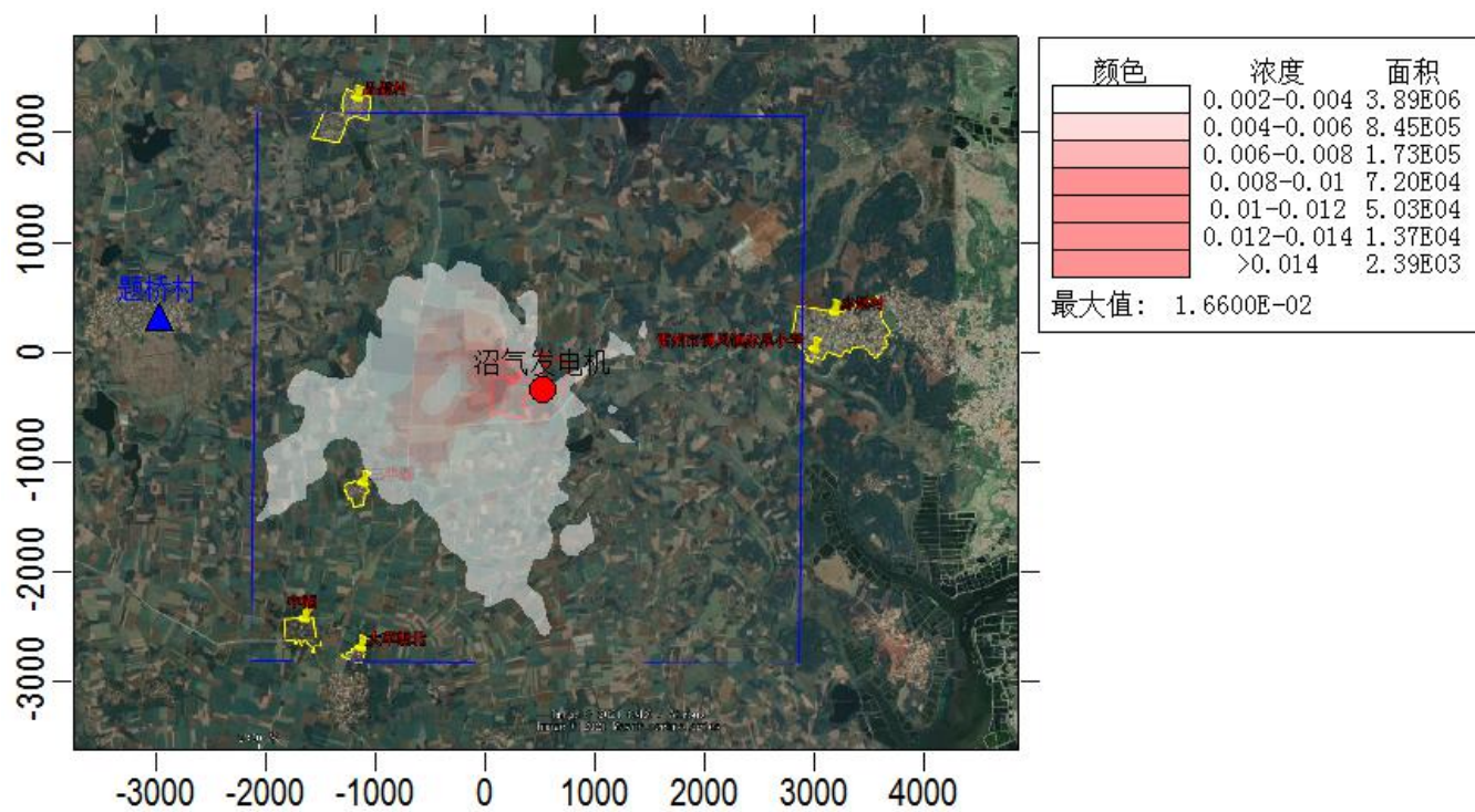
图 5.2-12 \text{NO}_2 1 小时平均浓度预测值分布图
