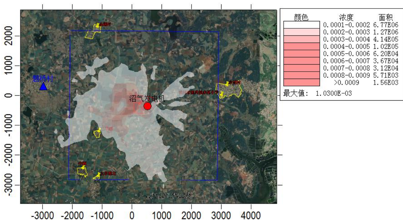
图 5.2-9 \text{SO}_2 小时平均浓度预测值分布图
