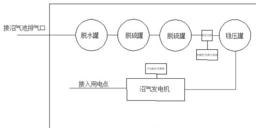
图 3.2-3 沼气发电系统流程图
