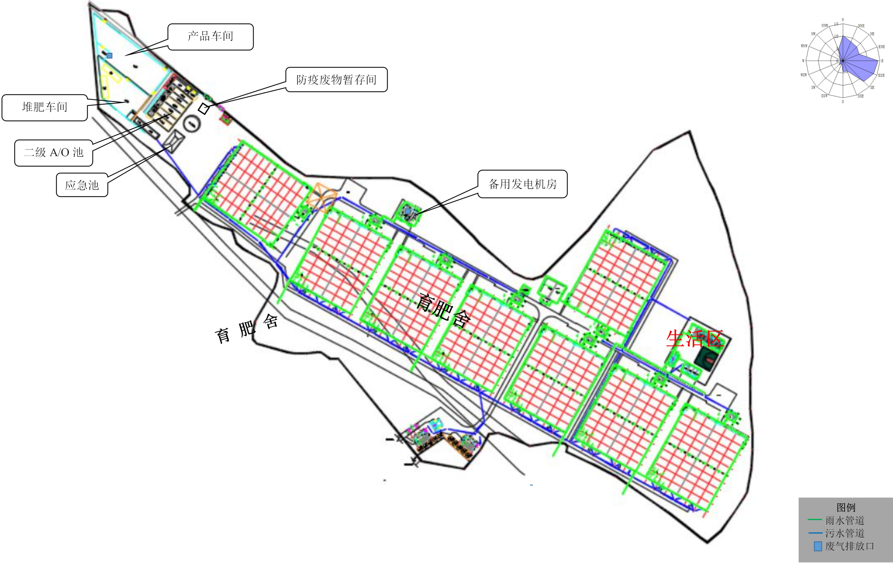
图 2.1-2 项目总平面布置图
