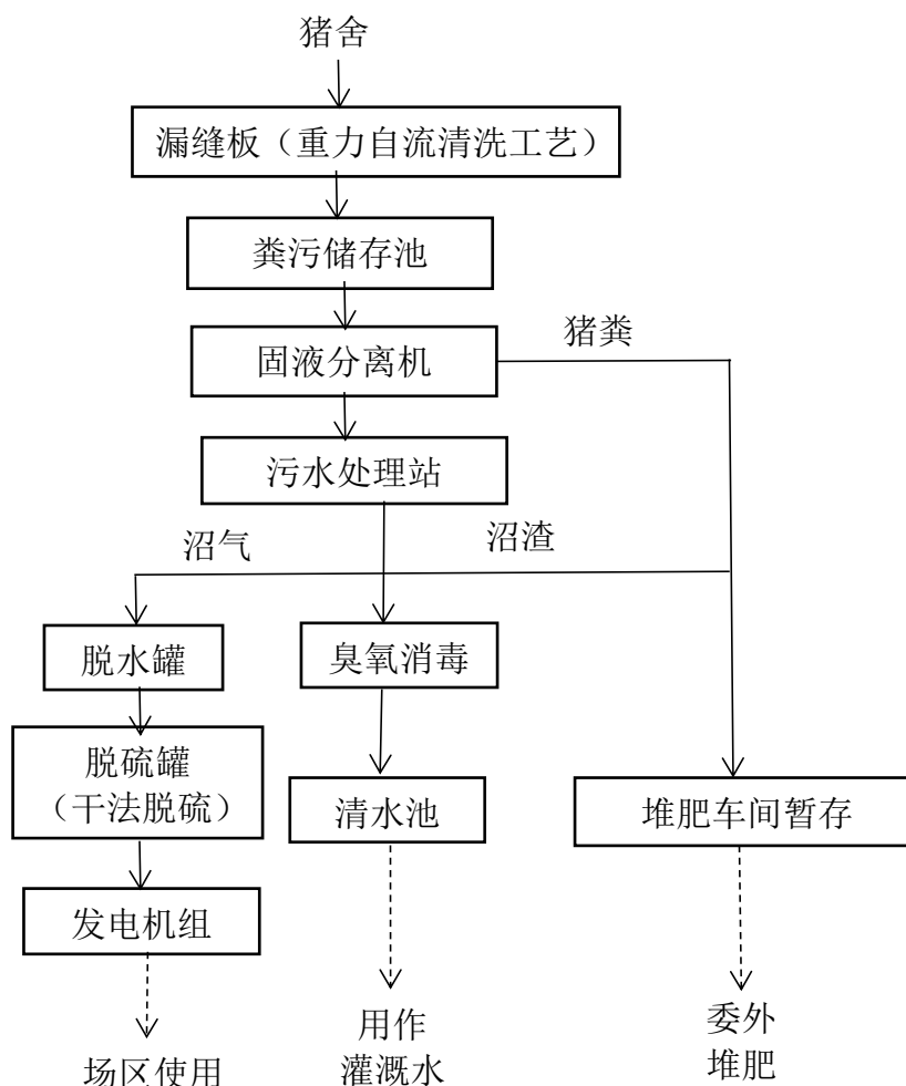
图 3.2-2 粪污处理及综合利用工艺图
