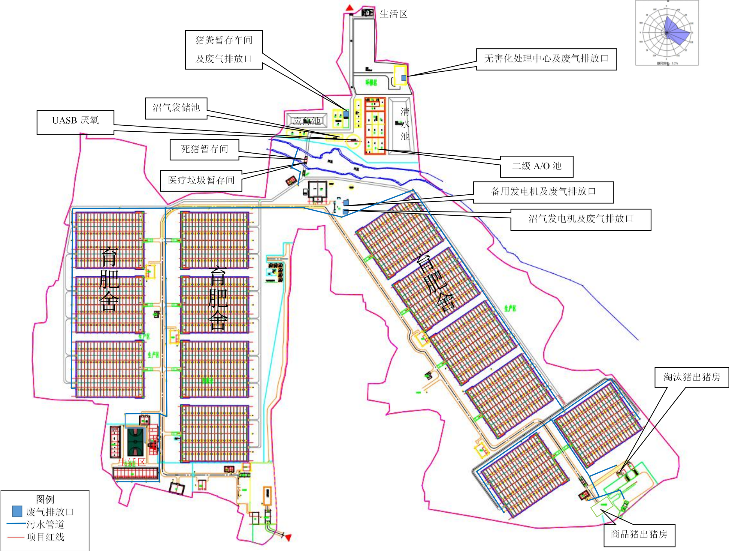
图 2.1-2 项目总平面布置图
