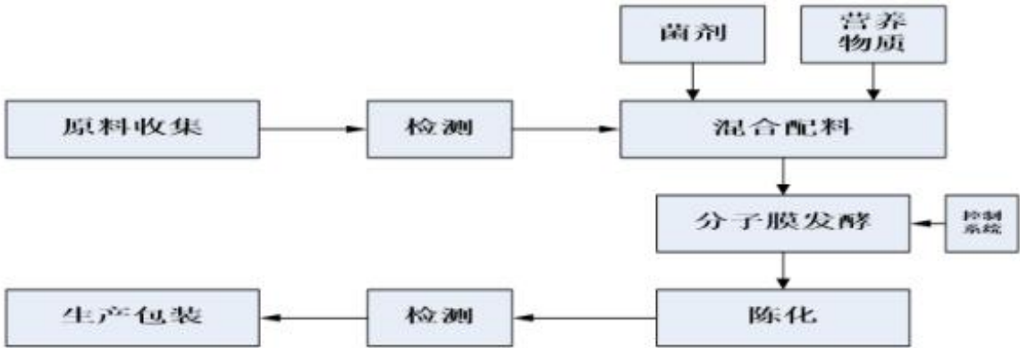
图 2: 原本“生物+气流膜”静态好氧堆肥发酵工艺流程
