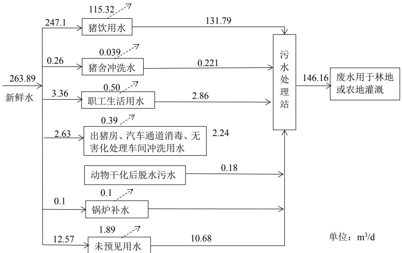
图 2.2-6 项目水平衡图
