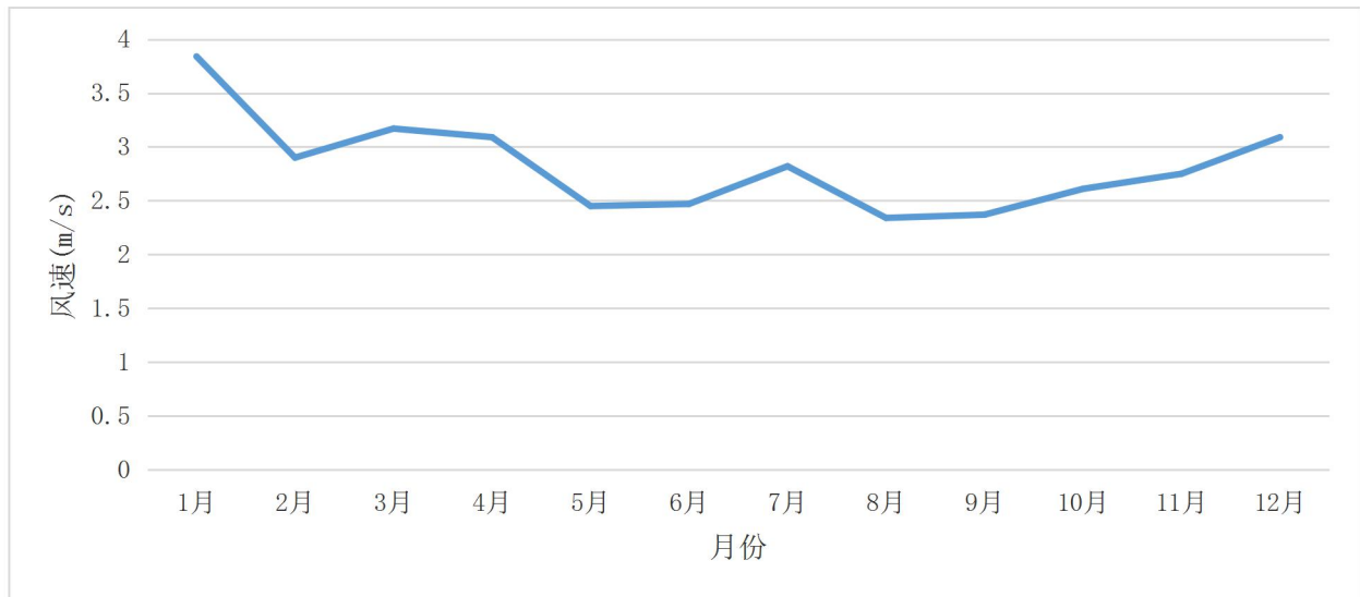
图 5.2-5 湛江市 2018 年各月平均风速变化曲线图
