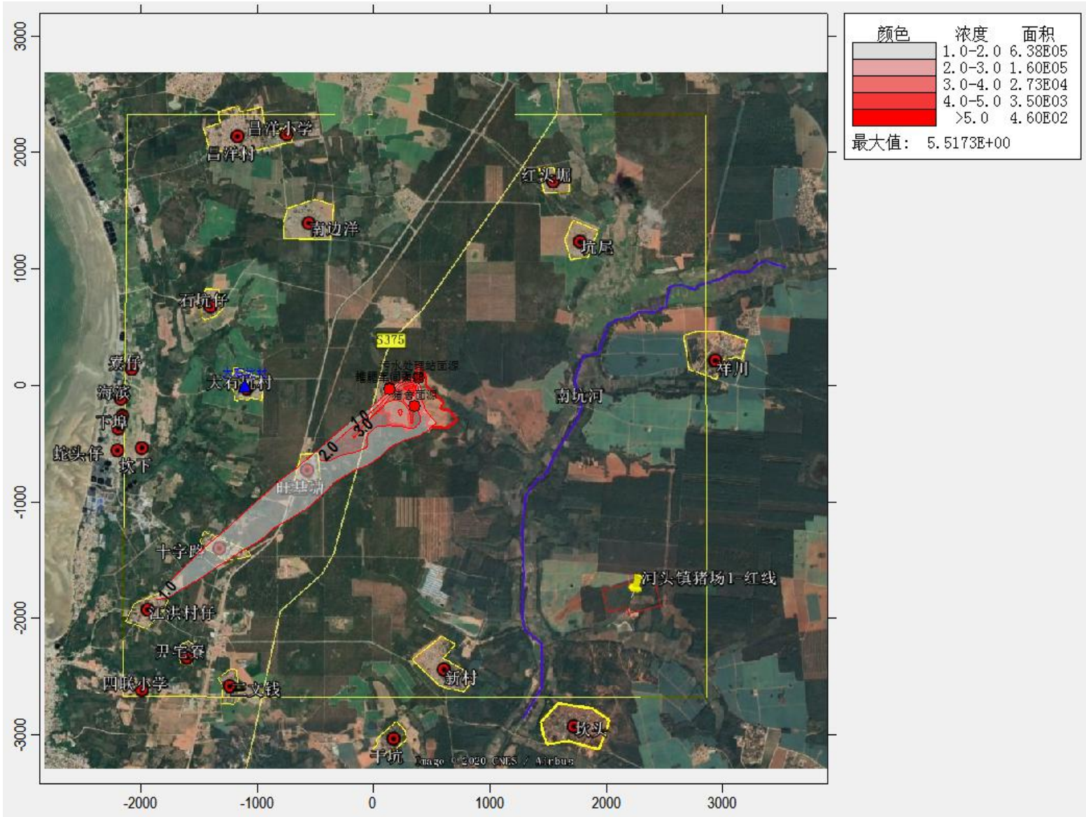
图 5.2-9 NH 3 小时浓度预测值分布图
