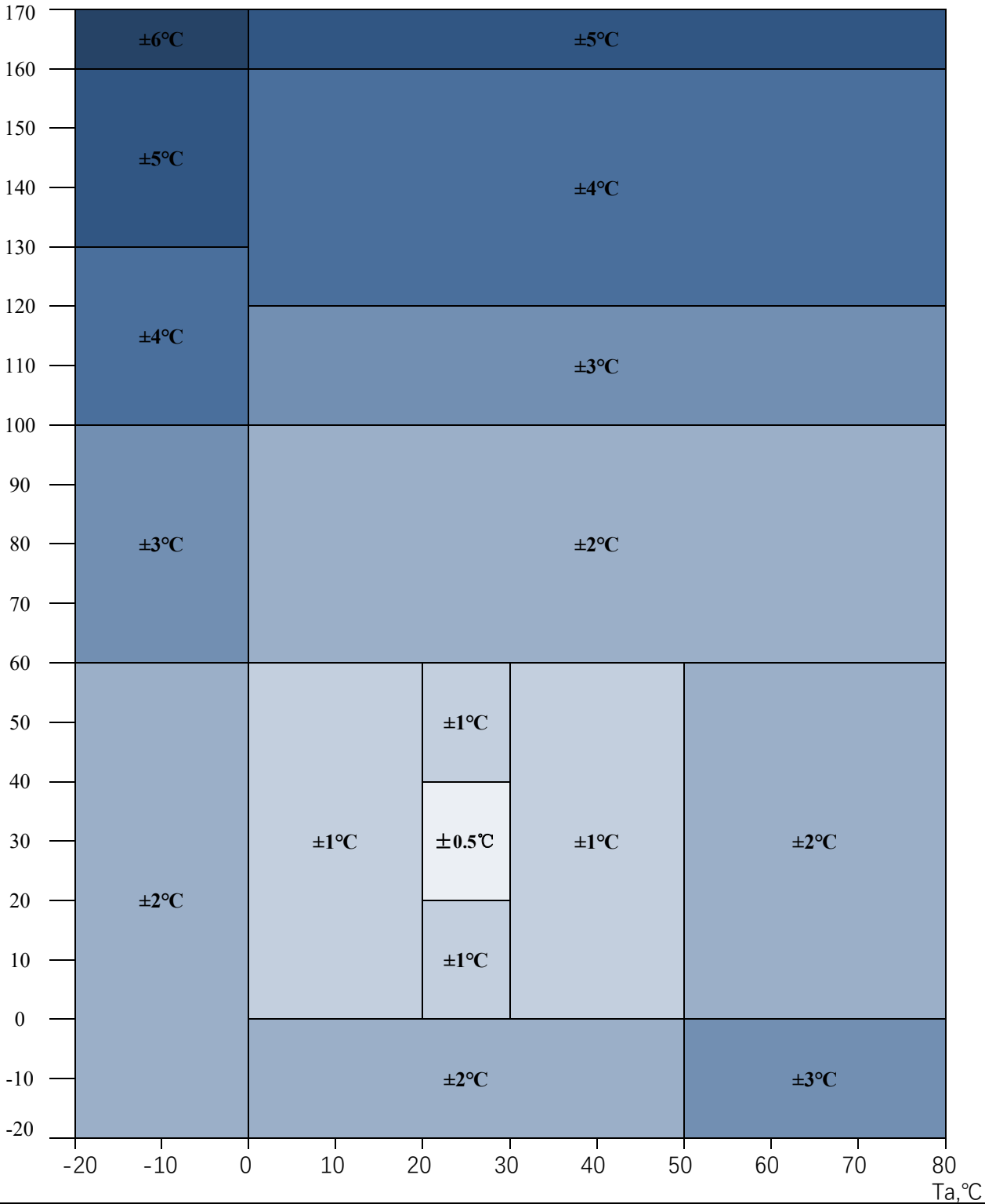
图 3.W-TRS-5.5DxI ( T_a, T_o ) 的标准精度
