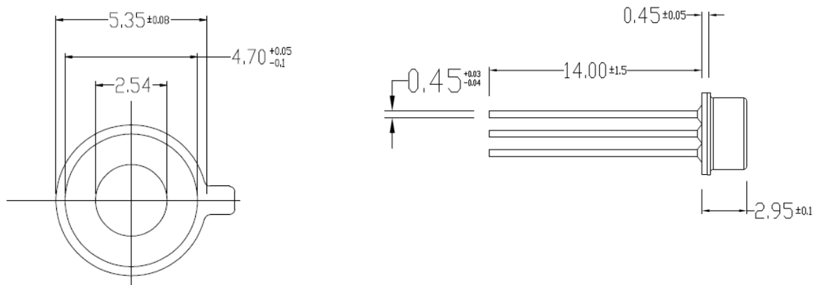
图 10 基体轮廓尺寸
